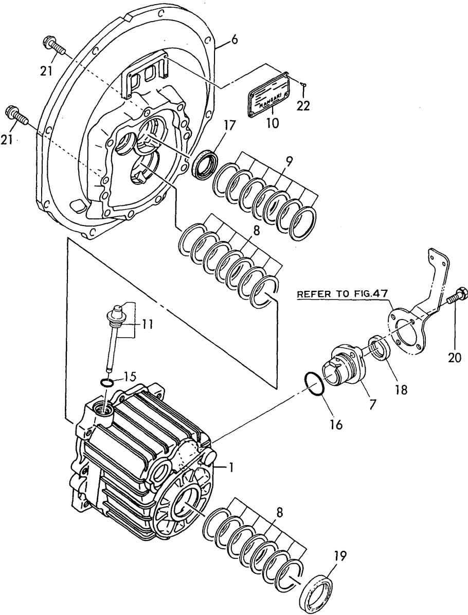
Fig. 43 クラッチケース CLUTCH HOUSING
