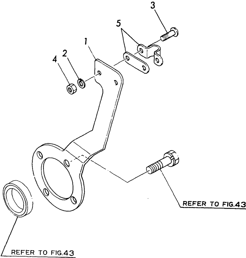
Fig.47 リモコンジュドウブ REMOTE CONTROL PASSIVE UNIT
