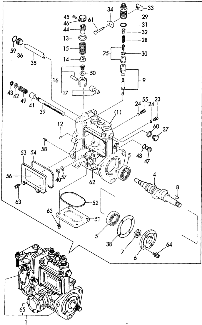
Fig. 17 FOフンシャポンプ FUEL INJECTION PUMP
