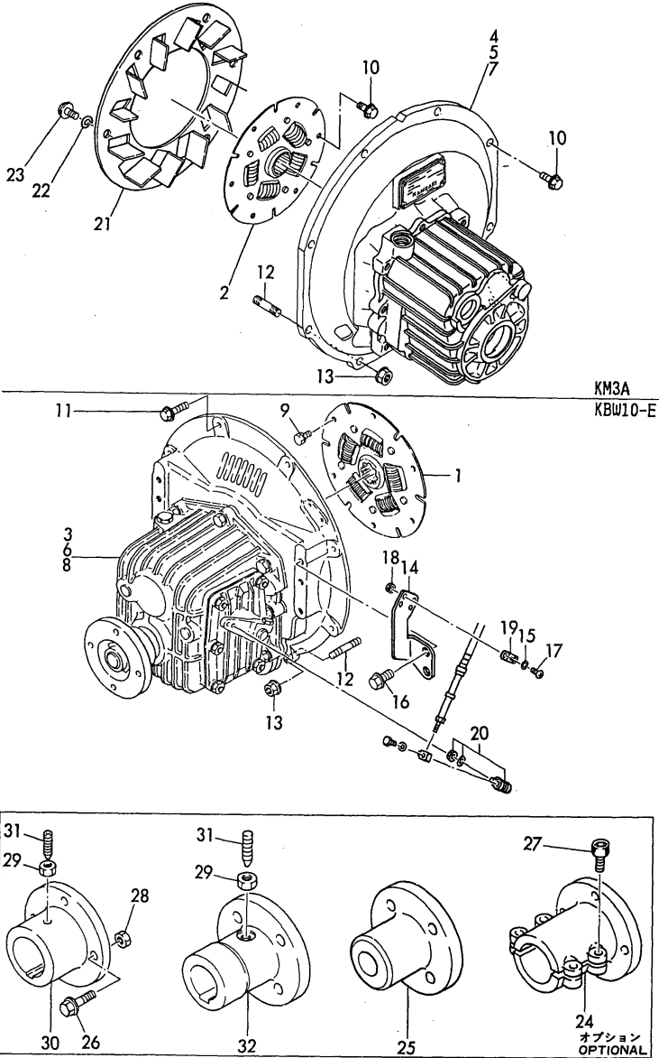
Fig.29 クラッチ CLUTCH
