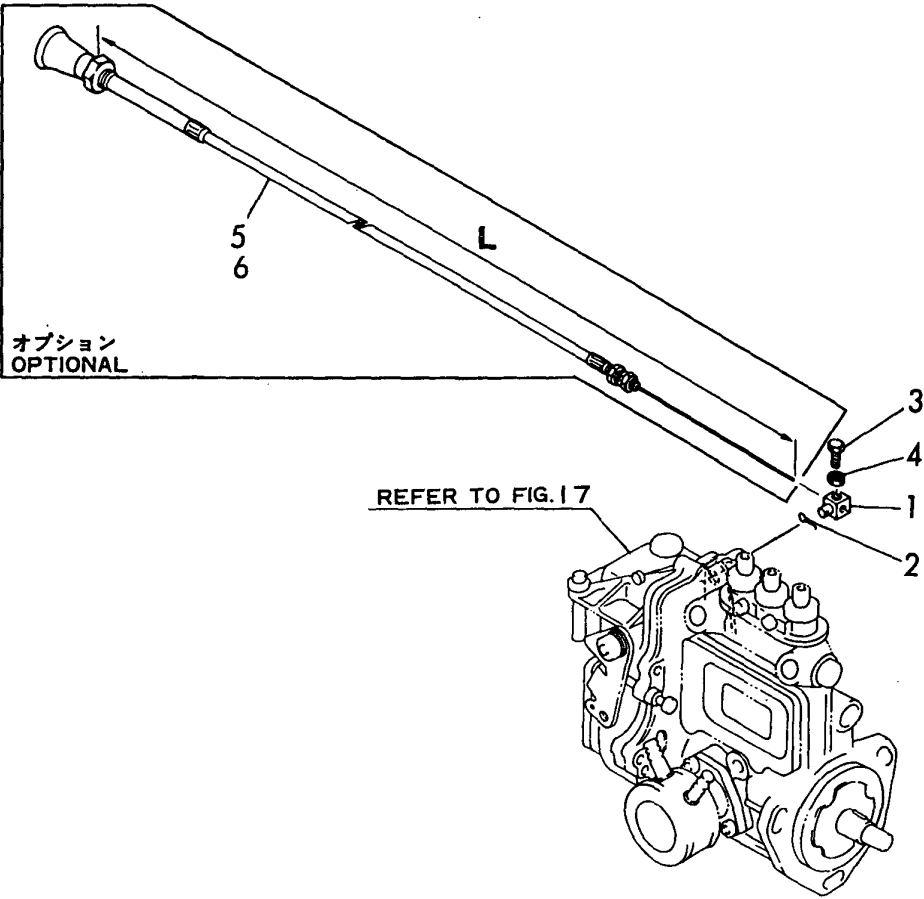
Fig. 23 キカンテイシソウチ ENGINE STOP DEVICE
