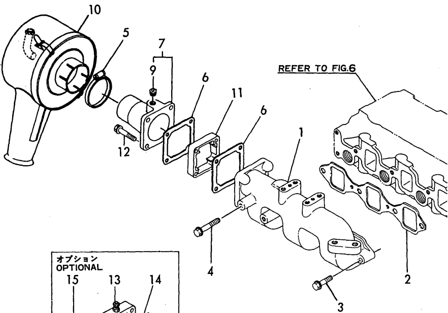
Fig.8 キュウキマニホールド SUCTION MANIFOLD
