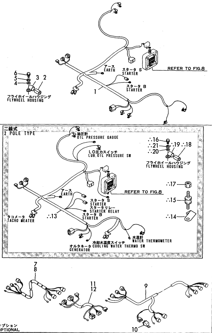
Fig.27 ワイヤハーネス WIRE HARNESS
