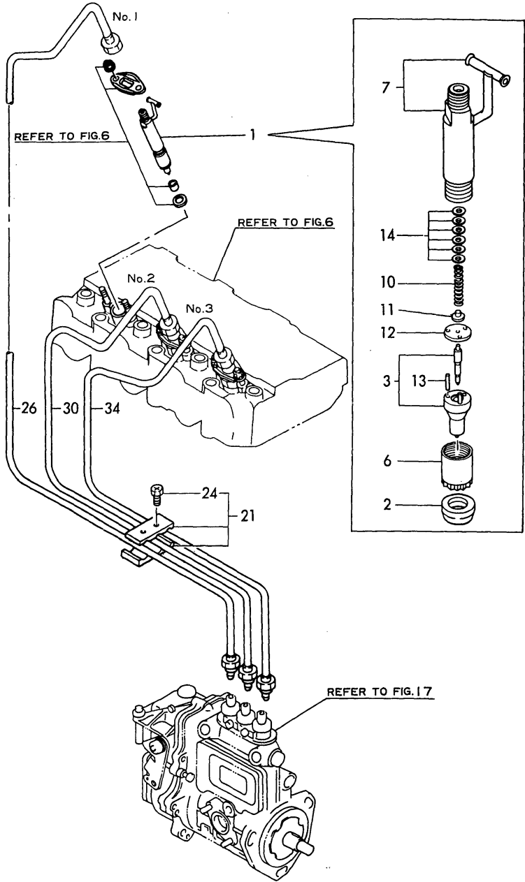
Fig. 19 FOフンシャパイプ & FOフンシャベン FUEL INJECTION LINE & INJECTION VALVE
