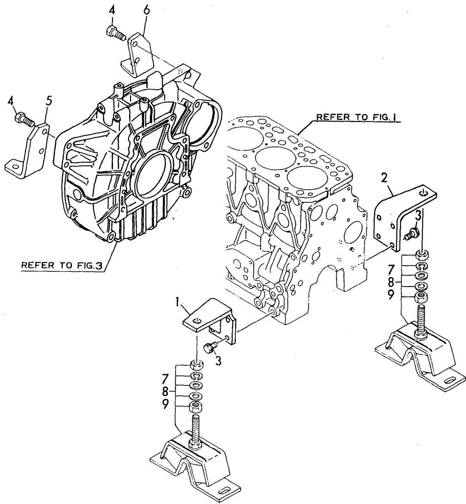
Fig.5 マウンティングフート ENGINE BRACKET
