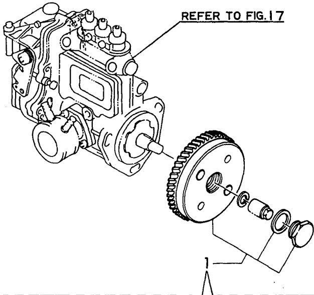
Fig. 20 タイマ TIMER
