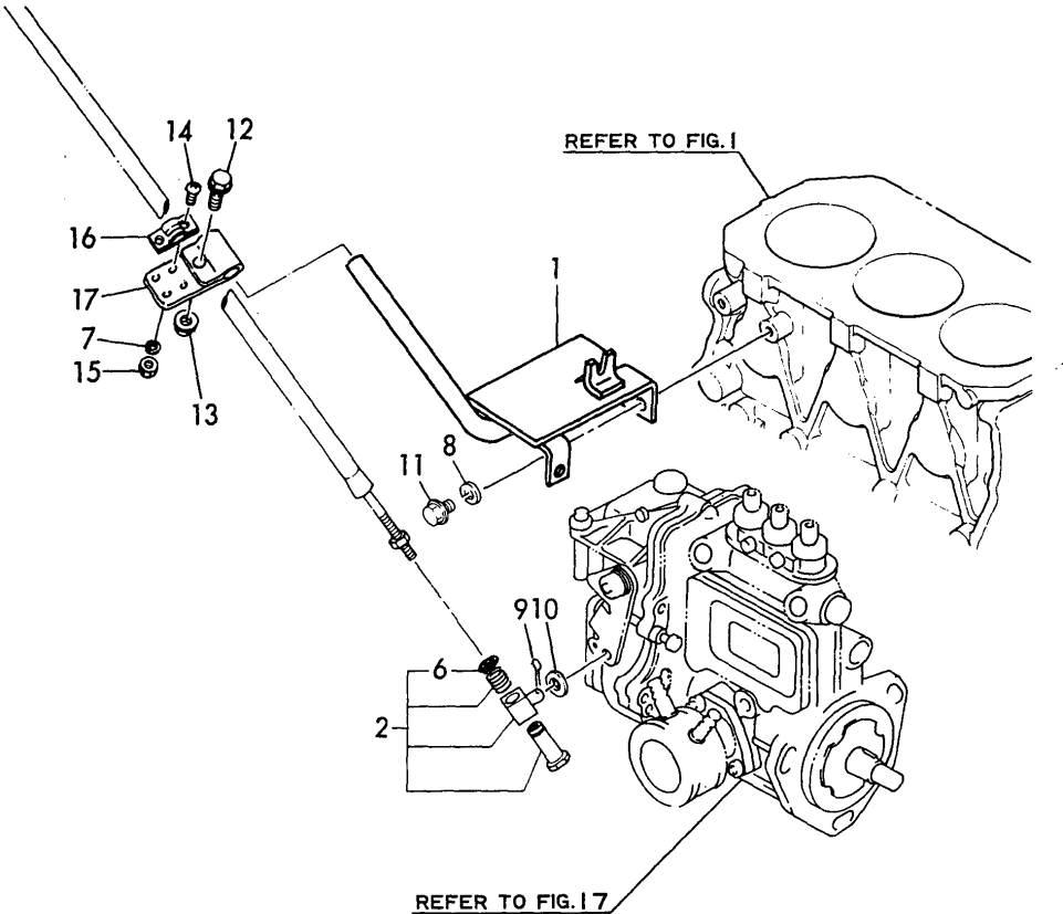
Fig. 24 スピードコントロールソウチ SPEED REMOTE CONTROL DEVICE
