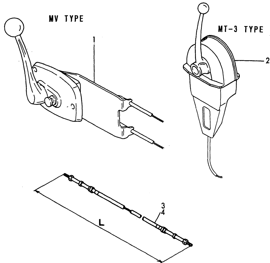
Fig. 38 リモコンソウチ(オプション) REMOTE CONTROL DEVICE (OPTIONAL)
