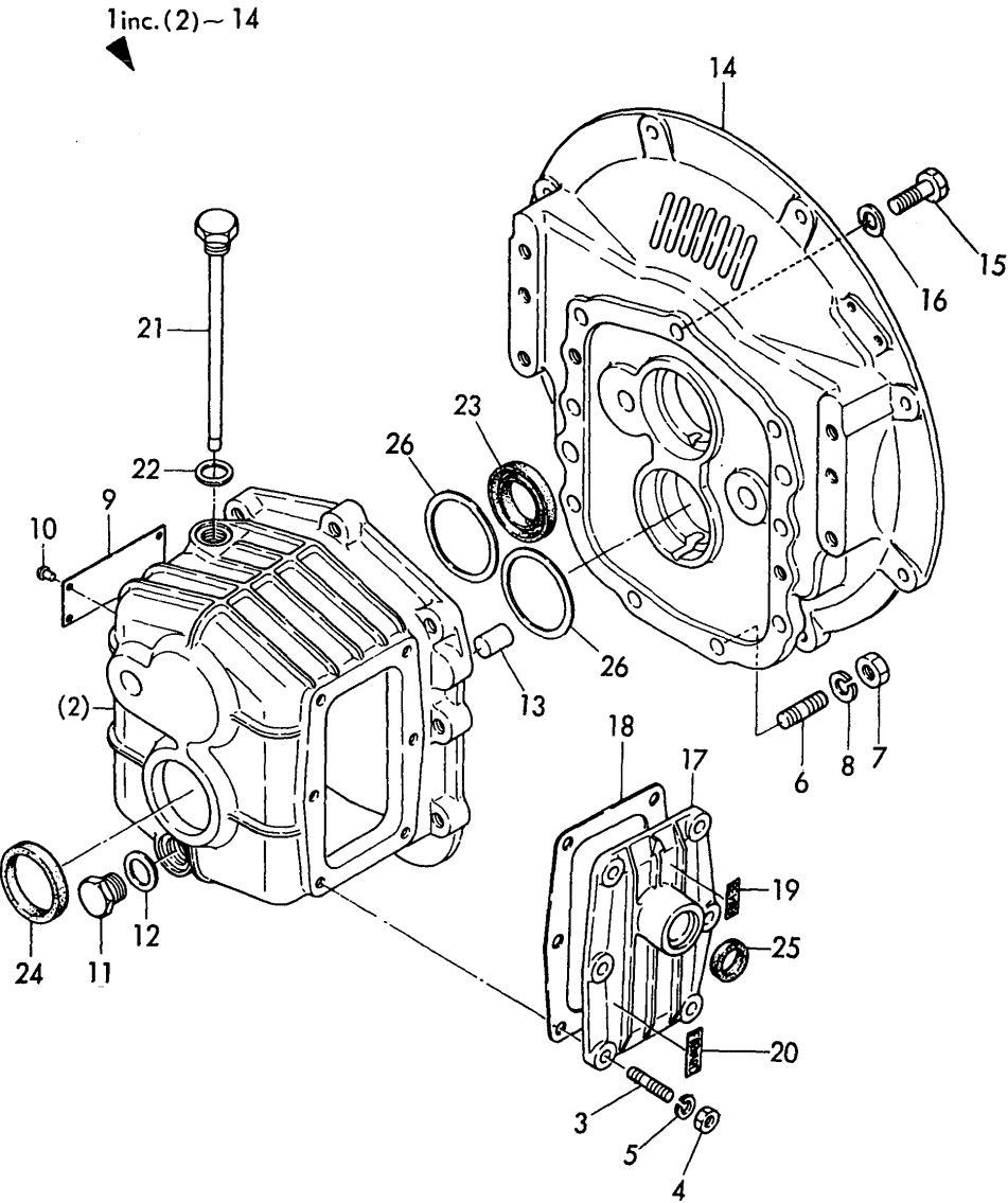
Fig.48 クラッチケース CLUTCH HOUSING
