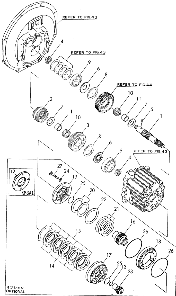
Fig.45 アウトプットシャフト OUTPUT SHAFT
