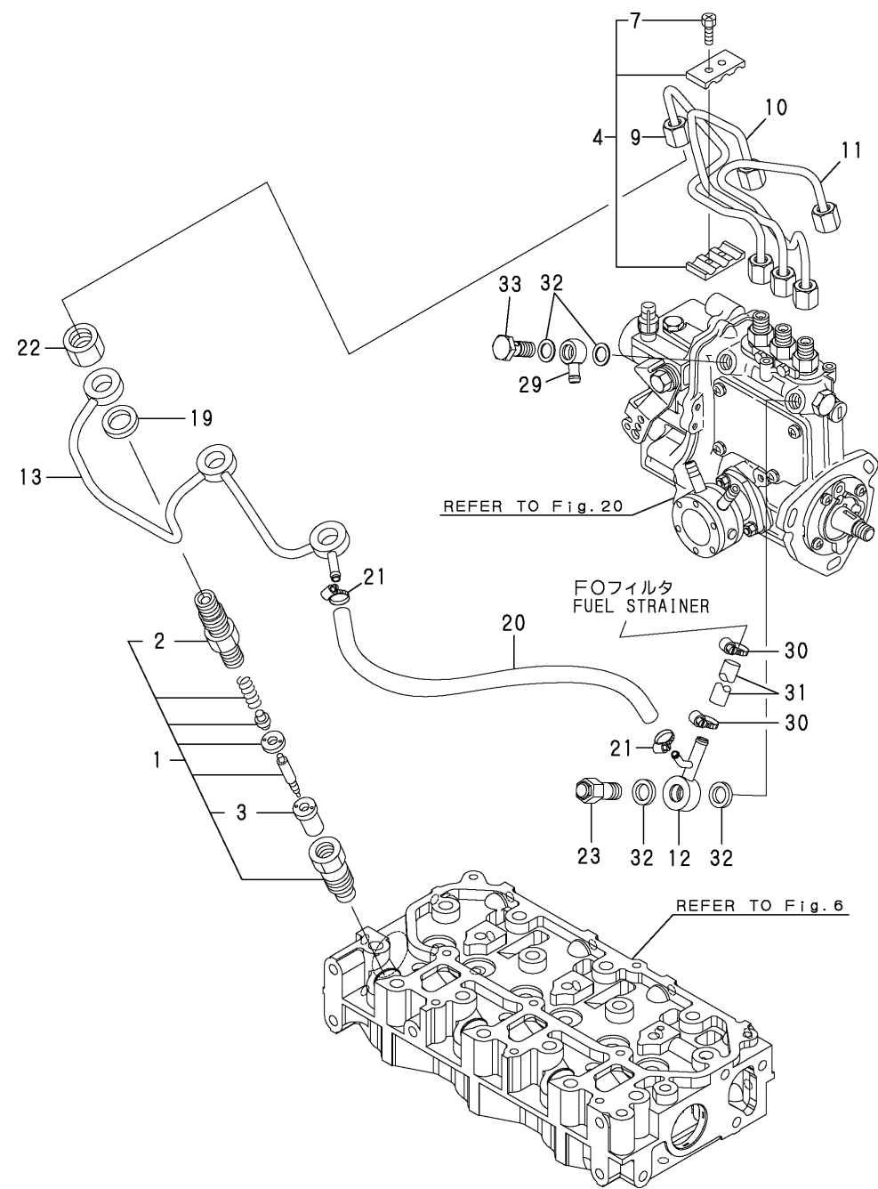
Fig.23.F.I.VALVE & F.I.PIPE
