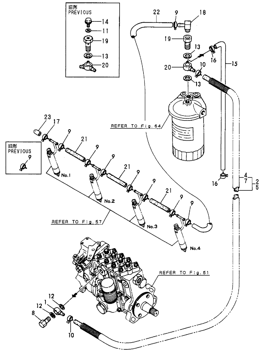
Fig.62 燃料戻しパイプ FUEL RETURN PIPE
