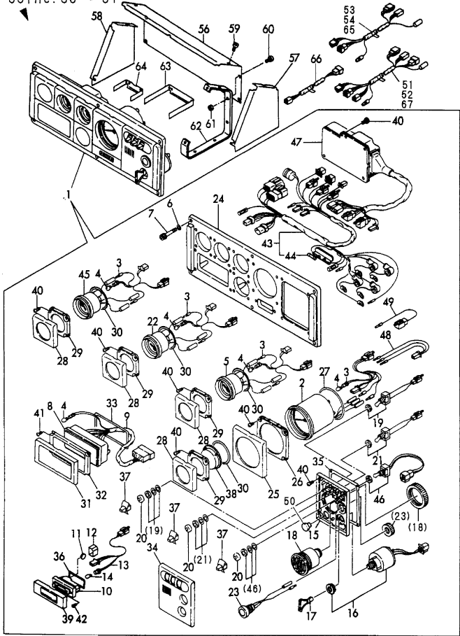
計器盤 (Dタイプ, 4LH-HTZ/DTZ) INSTRUMENT PANEL (D-TYPE, 4LH-HTZ/DTZ) 見出しNo. 55は、見出しNo. 56から61を含みます。 55inc. 56 ~ 61
