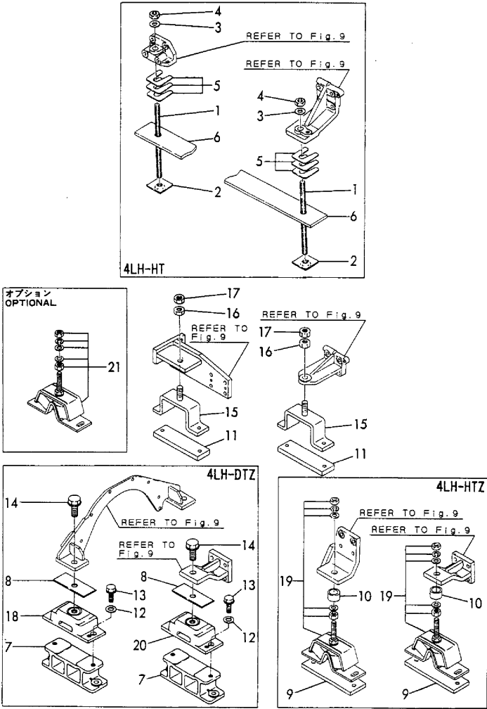
Fig. 10 機関取付台&基礎ボルト ENGINE BRACKET & FOUNDATION BOLT
