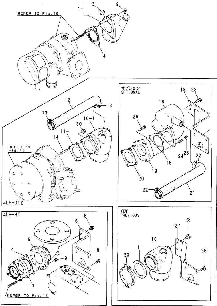
Fig. 14 ミキシングエルボ&排気バンド MIXING ELBOW & EXHAUST BEND
