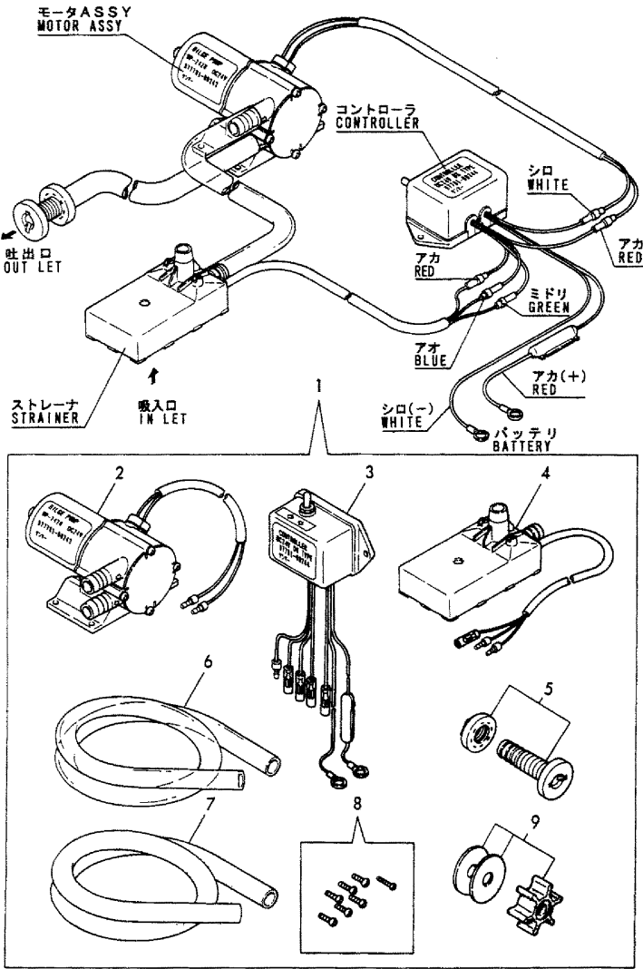
Fig.38 ビルジポンプ (DX, 旧形, オプション) BILGE PUMP (DX, PREVIOUS, OPT[ONAL])
