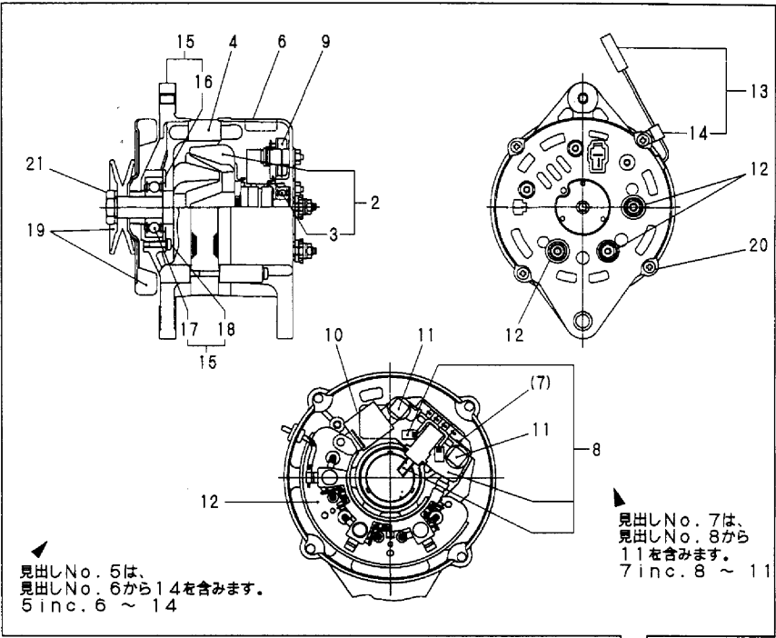
Fig.83 ジェネレータ (オプション) GENERATOR (OPTIONAL)
