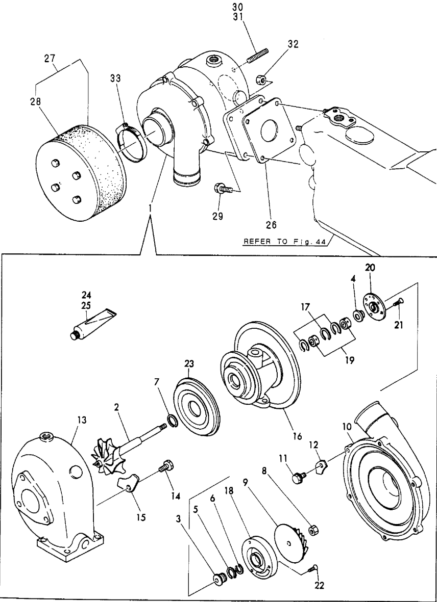
Fig. 17 タービン TURBOCHARGER
