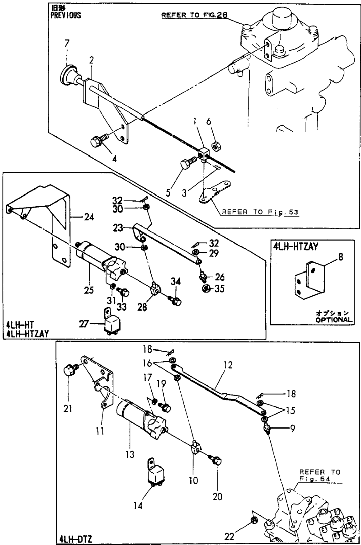
Fig.66 機関停止装置 ENGINE STOP DEVICE
