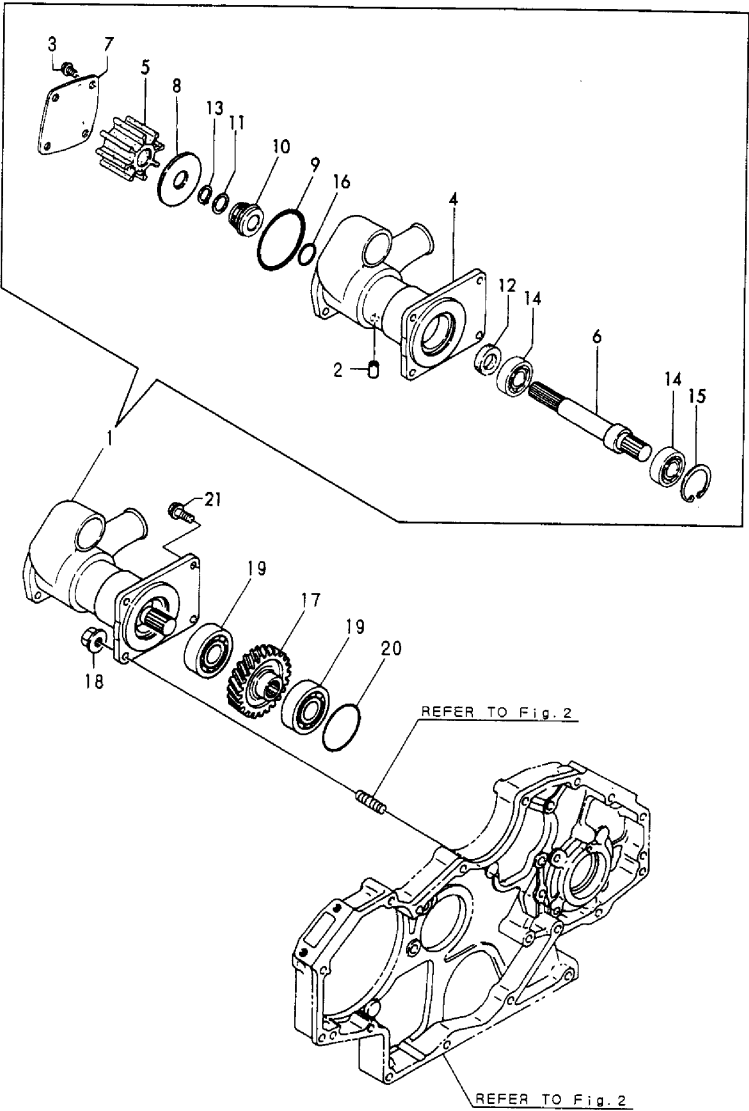
Fig.43 冷却水ポンプ (海水) COOLING SEA WATER PUMP
