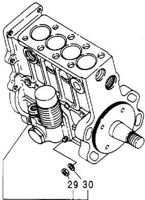
Fig.55 燃料フィードポンプ FUEL FEED PUMP
