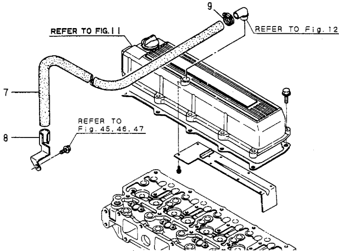
Fig.7 プリーザ BREATHER
