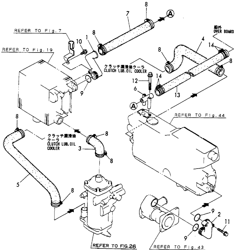
Fig.45 冷却水パイプ (海水, 4LH-HT) COOLING SEA WATER PIPE(4LH-HT)
