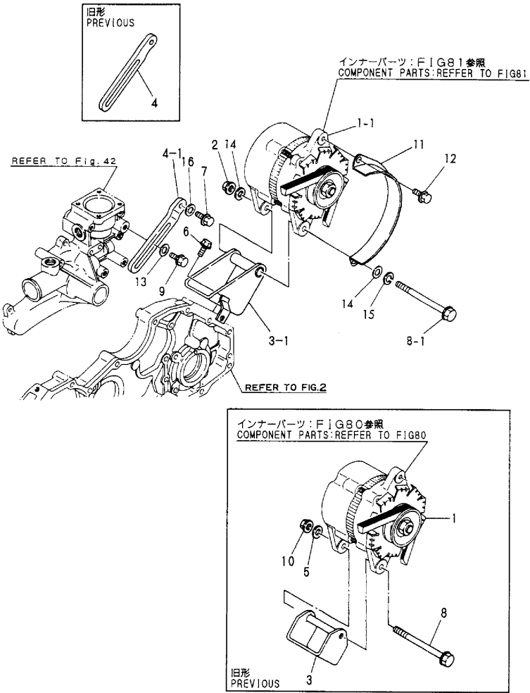
Fig.79 ジェネレータ (4LH-HT/HTZAY) GENERATOR (4LH-HT/HTZAY)
