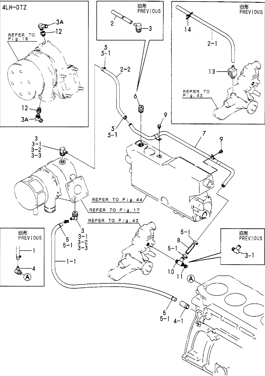
Fig.50 冷却水パイプ (清水, タービン) C. F. W. PIPE (TURBOCHARGER)
