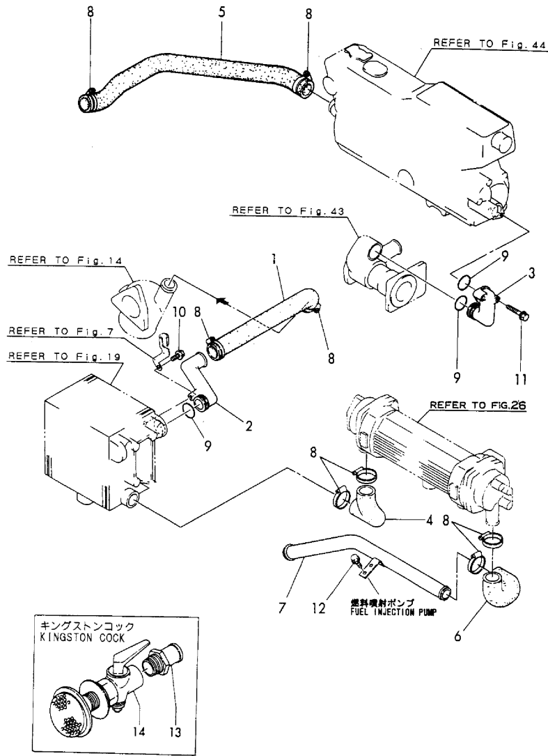
Fig.48 冷却水パイプ (海水, 4LH-DTZ) COOLING SEA WATER PIPE (4LH-DTZ)
