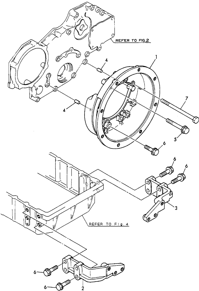
Fig.6 前部マウント FRONT BRACKET
