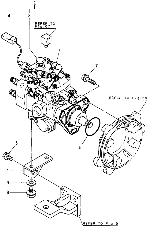
Fig.52 燃料噴射ポンプ (4LH-HTZ) FUEL INJECTION PUMP (4LH-HTZ)
