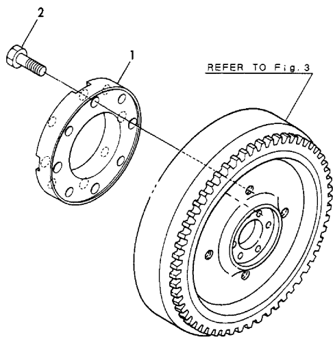
Fig.22 継手&ダンパーディスク COUPLING & DUMPER DISK
