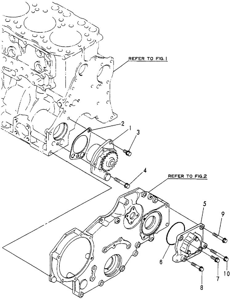
Fig.25 潤滑油ポンプ LUB.OIL PUMP
