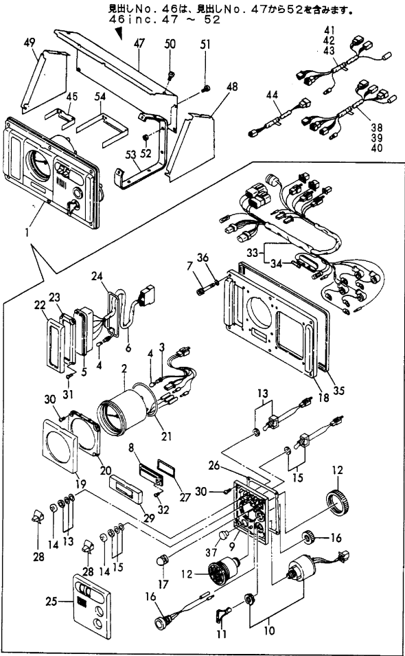
計器盤 (Bタイプ, オプション, 4LH-HTZ/DTZ) INSTRUMENT PANEL (B-TYPE,OPTIONAL, 4LH-HTZ/DTZ)
