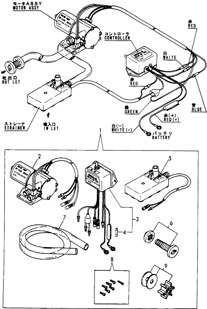
Fig.40 ビルジポンプ (DX, 旧形, オプション) BILGE PUMP (DX, PREVIOUS, OPTIONAL)
