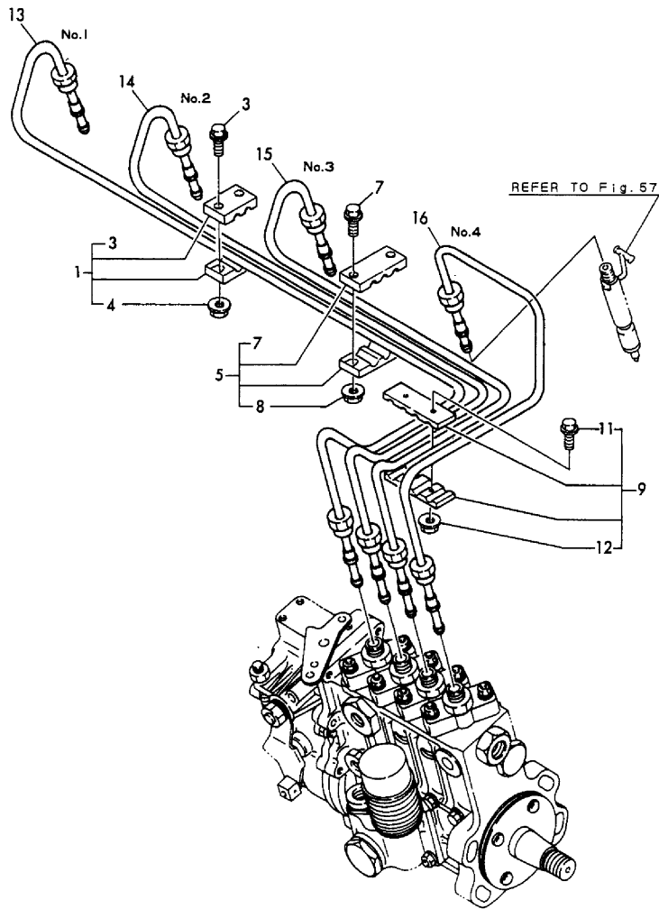
Fig.58 燃料噴射パイプ FUEL INJECTION PIPE
