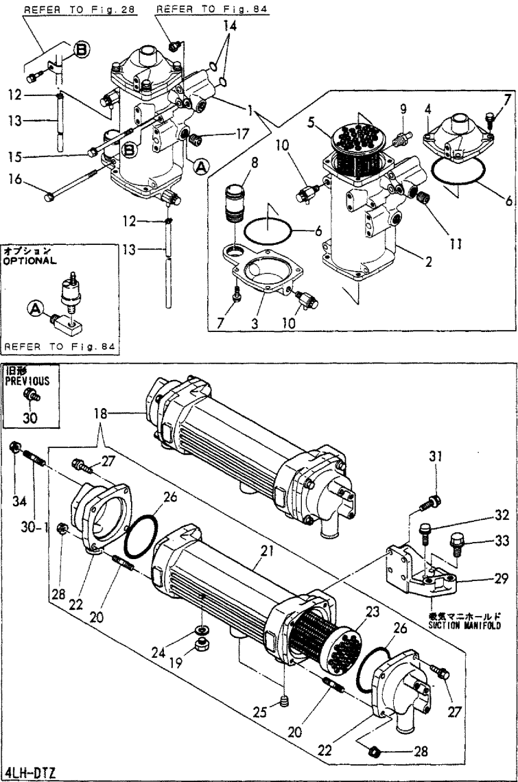
Fig.26 潤滑油クーラ LUB.OIL COOLER
