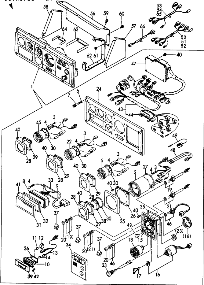
Fig. 92 計器盤 (Dタイプ, 4LH-HTZAY) INSTRUMENT PANEL (D-TYPE, 4LH-HTZAY) 見出しNo. 55は、見出しNo. 56から61を含みます。 55 inc. 56 ~ 61
