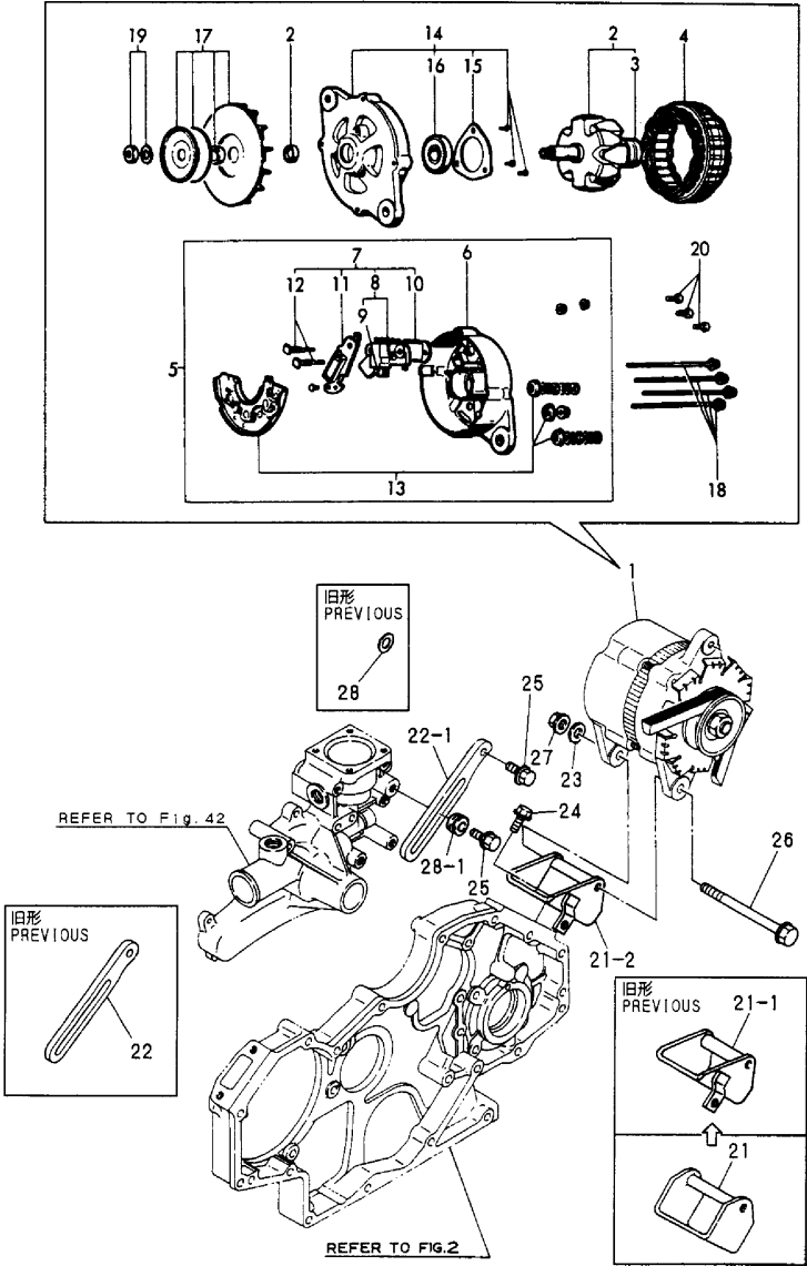
Fig.82 ジェネレータ (4LH-HTZ/DTZ) GENERATOR (4LH-HTZ/DTZ)
