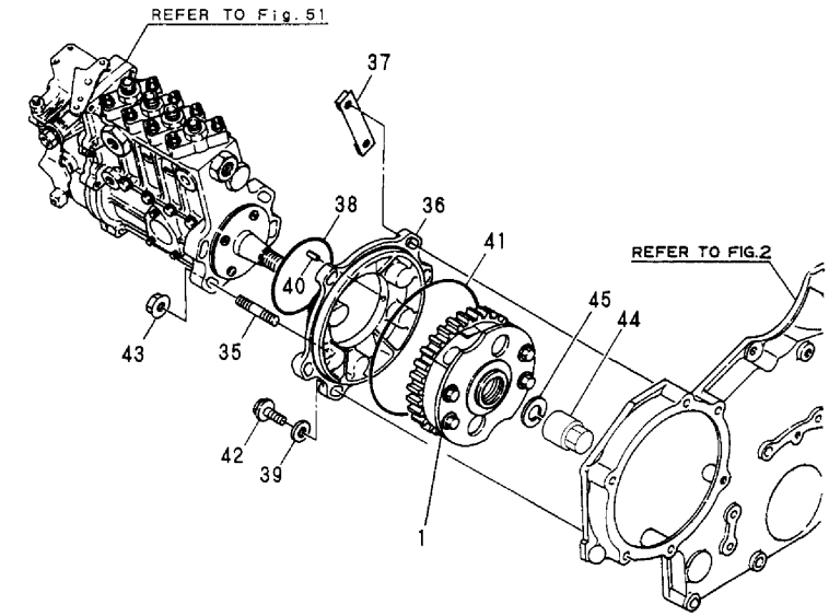
Fig.56 タイマ TIMER
