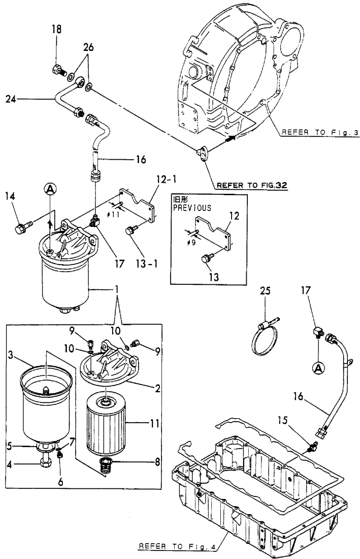
Fig.34 潤滑油パイプ (バイパス) LUB.OIL PIPE (BY-PASS)
