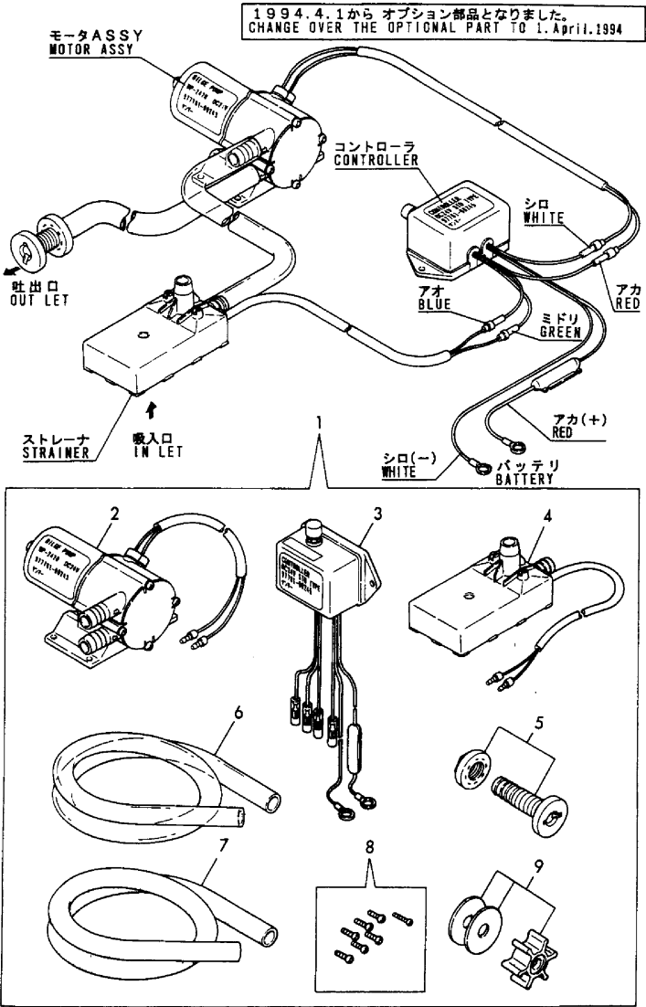
Fig.37 ビルジポンプ (STD, 旧形, オプション) BILGE PUMP (STD, PREVIOUS, OPTIONAL)
