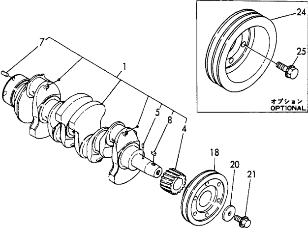
Fig.21 クランクシャフト CRANKSHAFT
