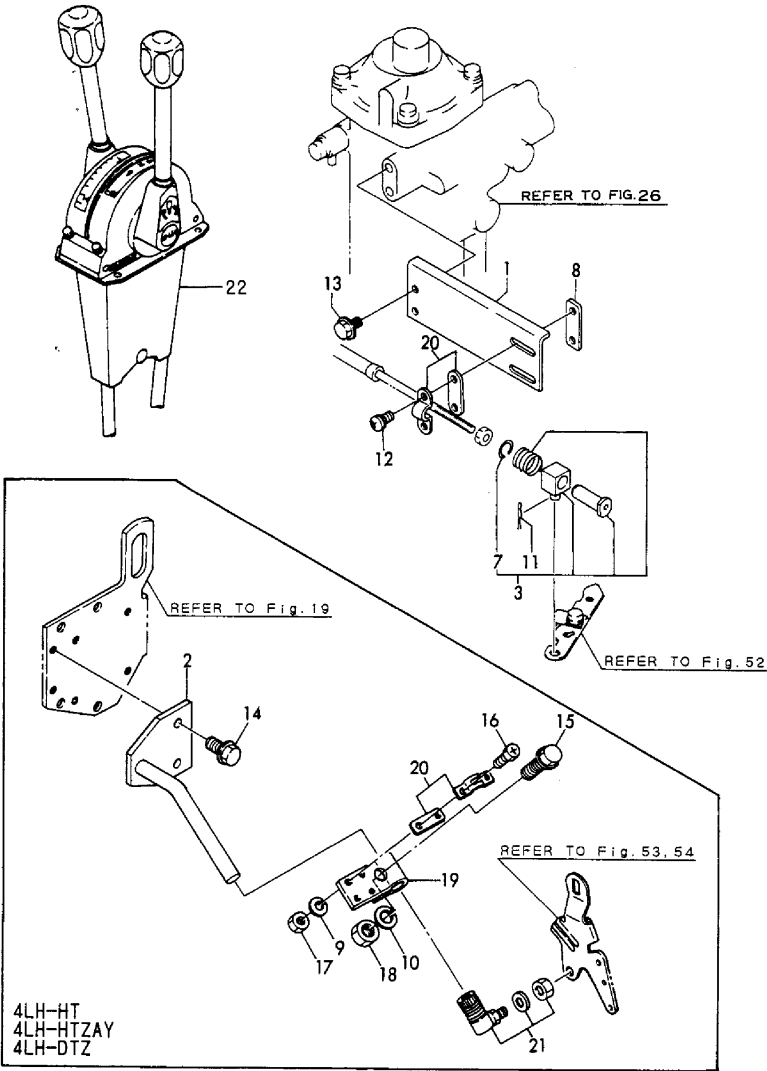
Fig.67 ケーブル支持台 CABLE SUPPORT
