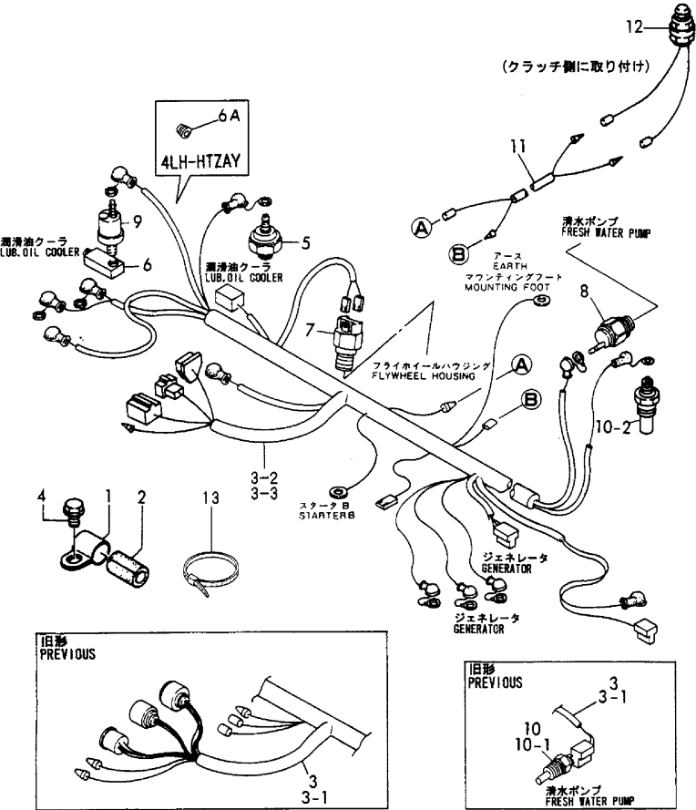
Fig.84 ワイヤーハーネス&センサ (4LH-HT/HTZAY) WIRE HARNESS & SENSOR(4LH-HT/HTZAY)
