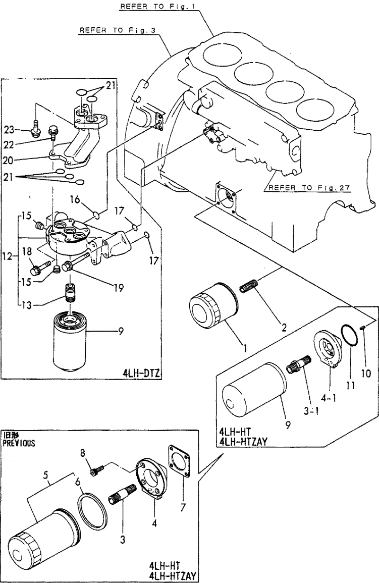
Fig.29 潤滑油フィルタ LUB.OIL STRAINER
