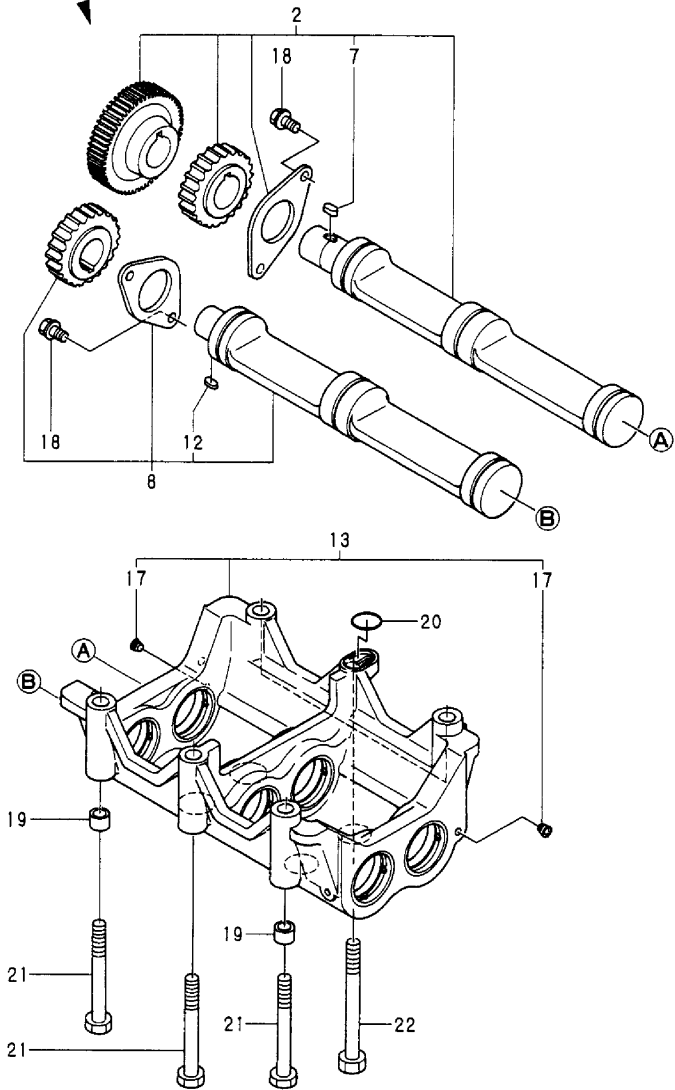
Fig.24 バランサ BALANCER
