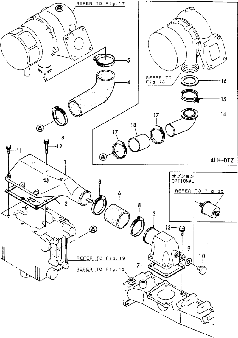
Fig.20 エアダクト AIR DUCT
