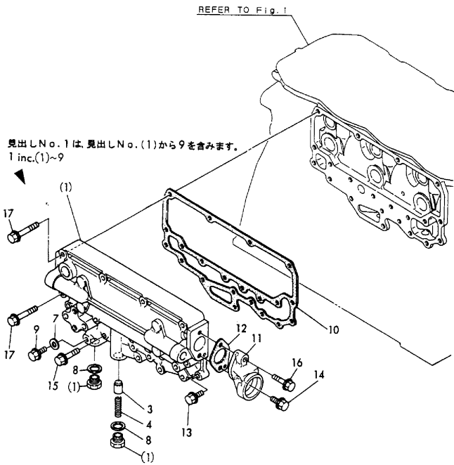
Fig.27 潤滑油クーラケース LUB.OIL COOLER HOUSING
