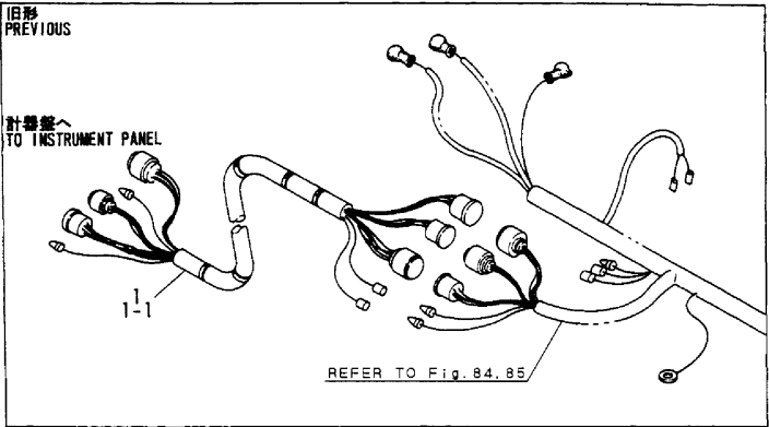
Fig.86 エクステンションコード EXTENSION WIRE
