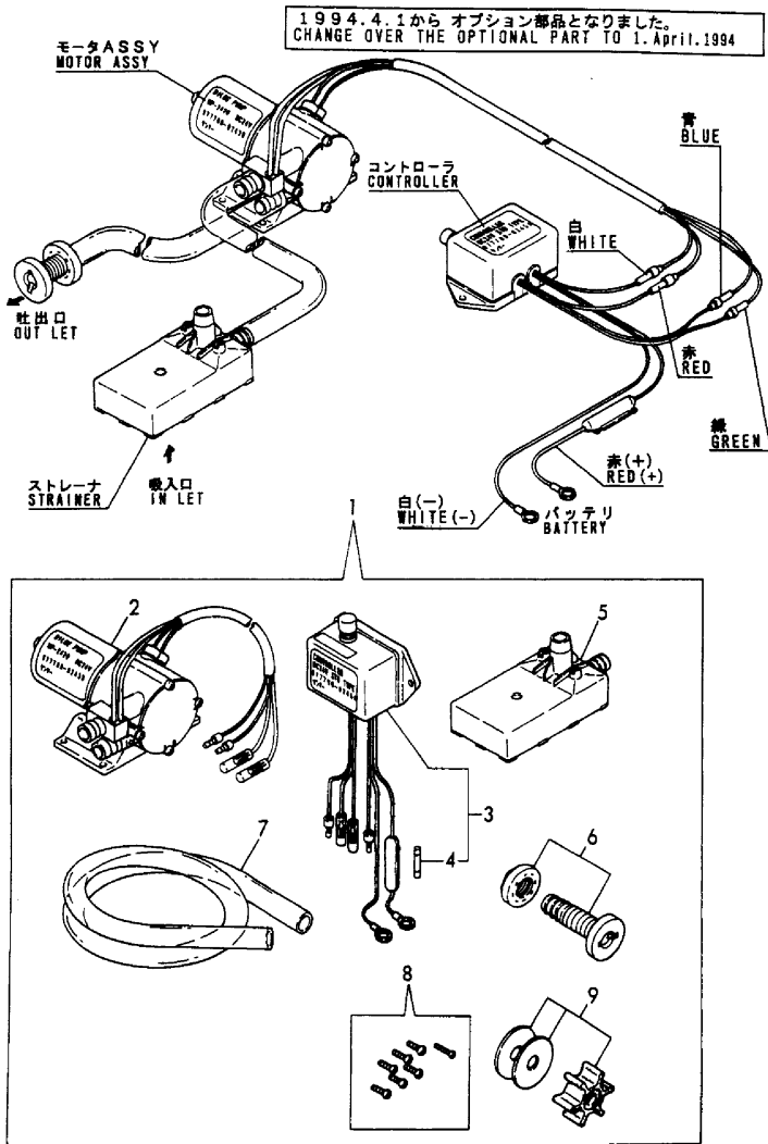
Fig.39 ビルジポンプ (STD, 旧形, オプション) BILGE PUMP (STD, PREVIOUS, OPTIONAL)
