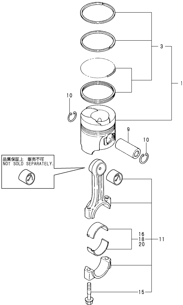
Fig. 14 ピストン&コネクティングロッド PISTON & CONNECTING ROD
