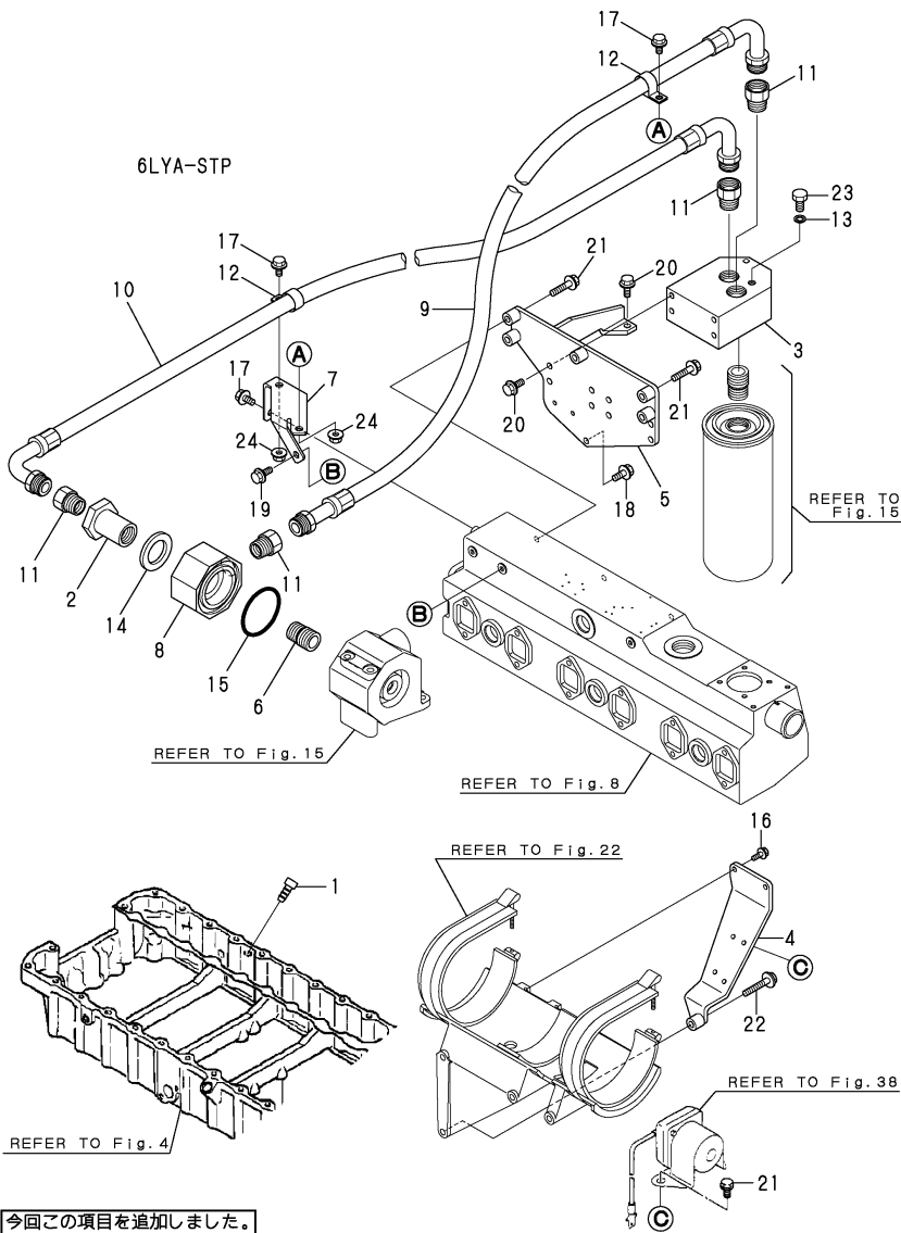
リモート潤滑油フィルタ (オプション) REMOTE LUB.OIL STRAINER (OPTIONAL)
