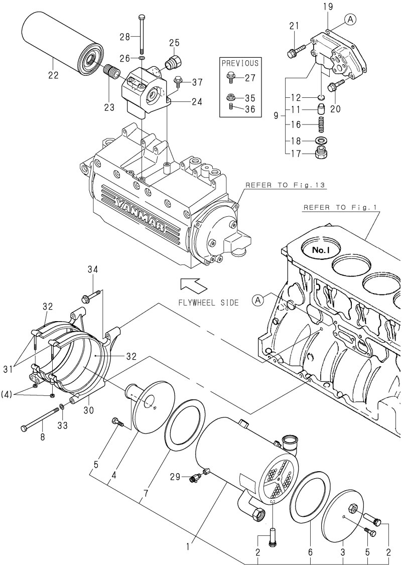
Fig. 15 LUB.OIL COOLER & LUB.OIL STRAINER
