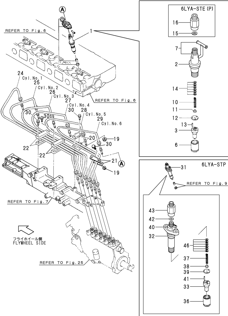
Fig.29 燃料噴射パイプ&燃料噴射弁 F.I.PIPE & F.I.VALVE
