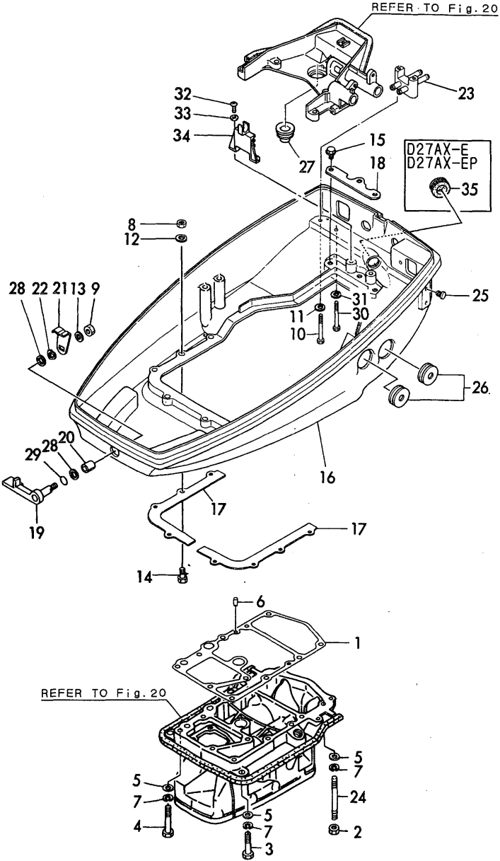
Fig.19 ボトムカウリング&接続部品 BOTTOM COWLING & CONNECTING PART
