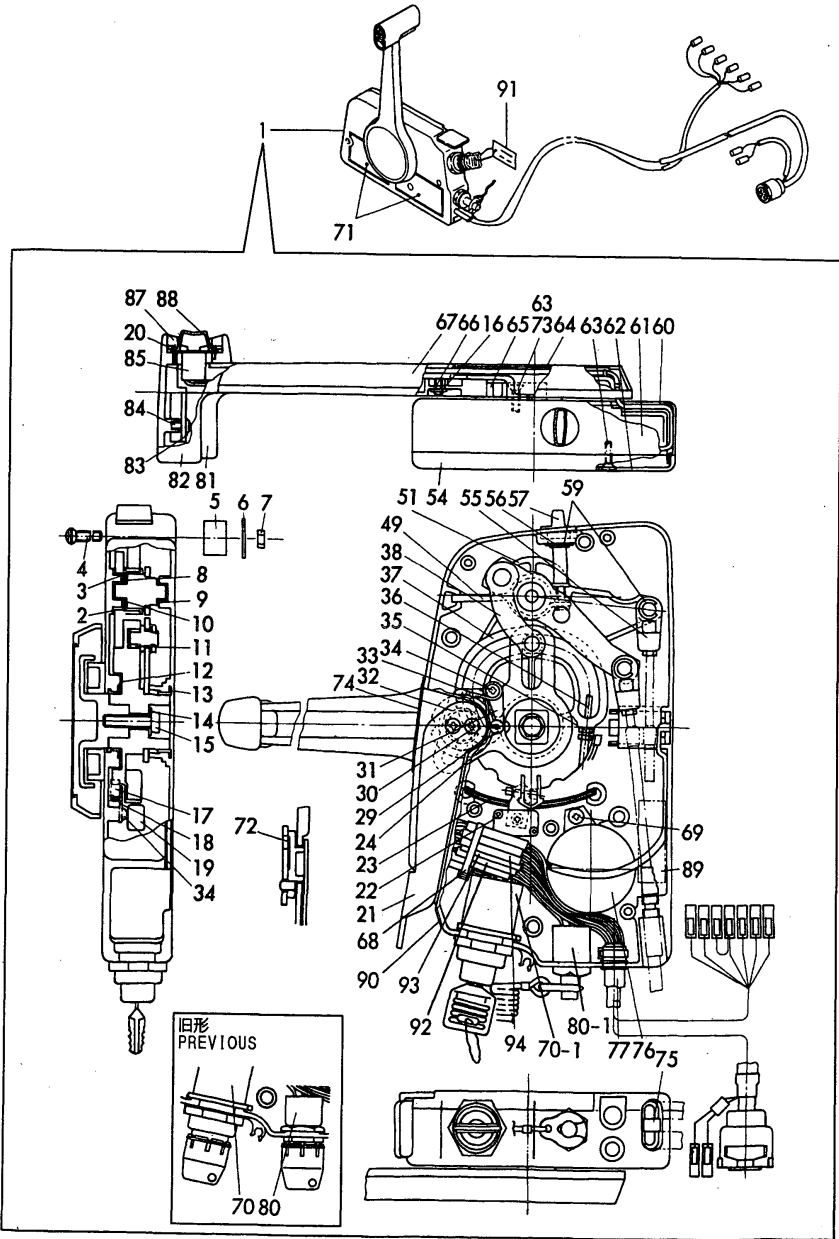
Fig.26 NA12 リモートコントロールハンドル (オプション) NA12 REMOTE CONTROL HANDLE (OPTIONAL)
