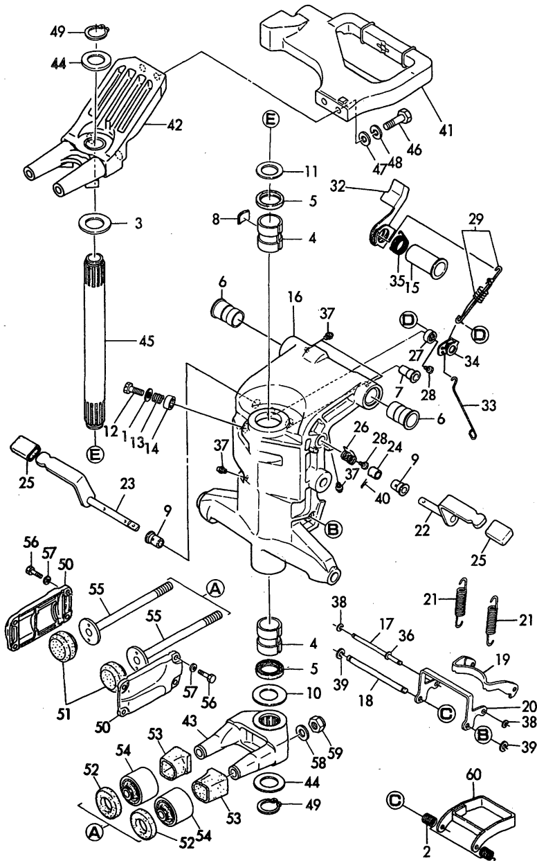
Fig. 15 スイベル/ステアリングブラケット SWIVEL/STEERING BRACKET
