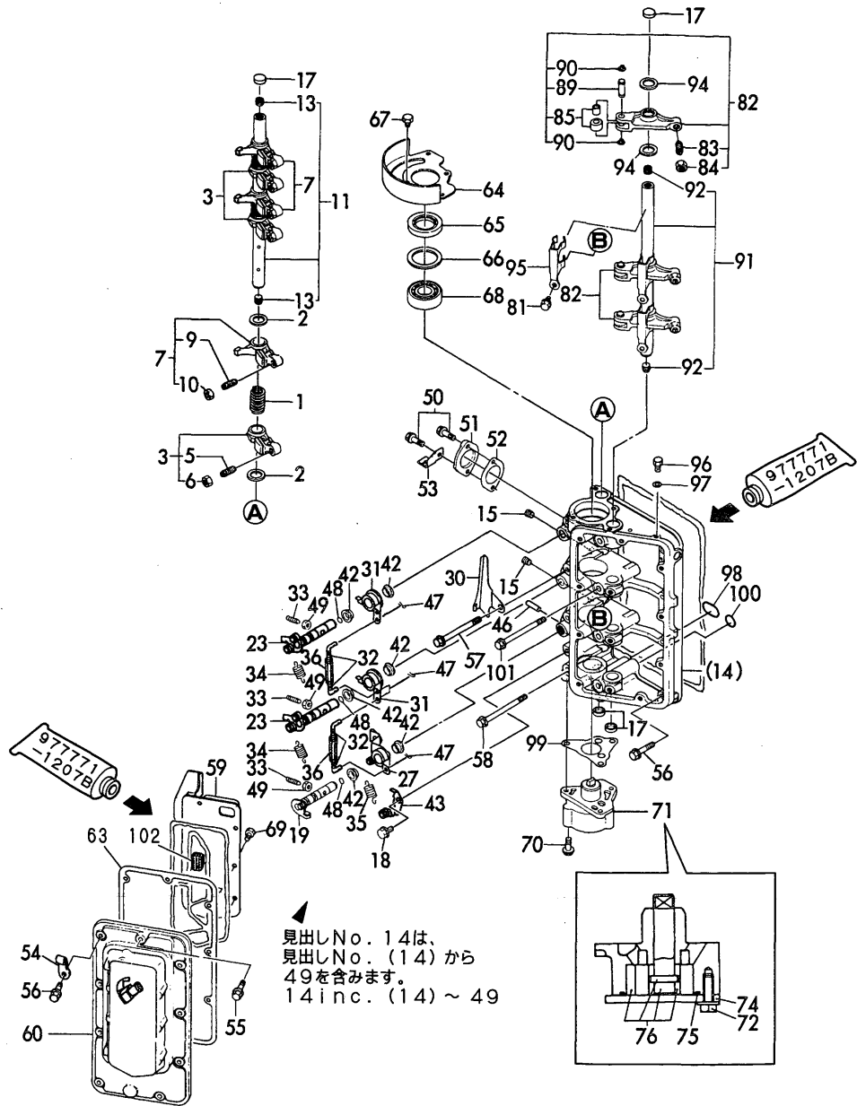
Fig.4 ボンネット&潤滑油ポンプ BONNET & LUB.OIL PUMP
