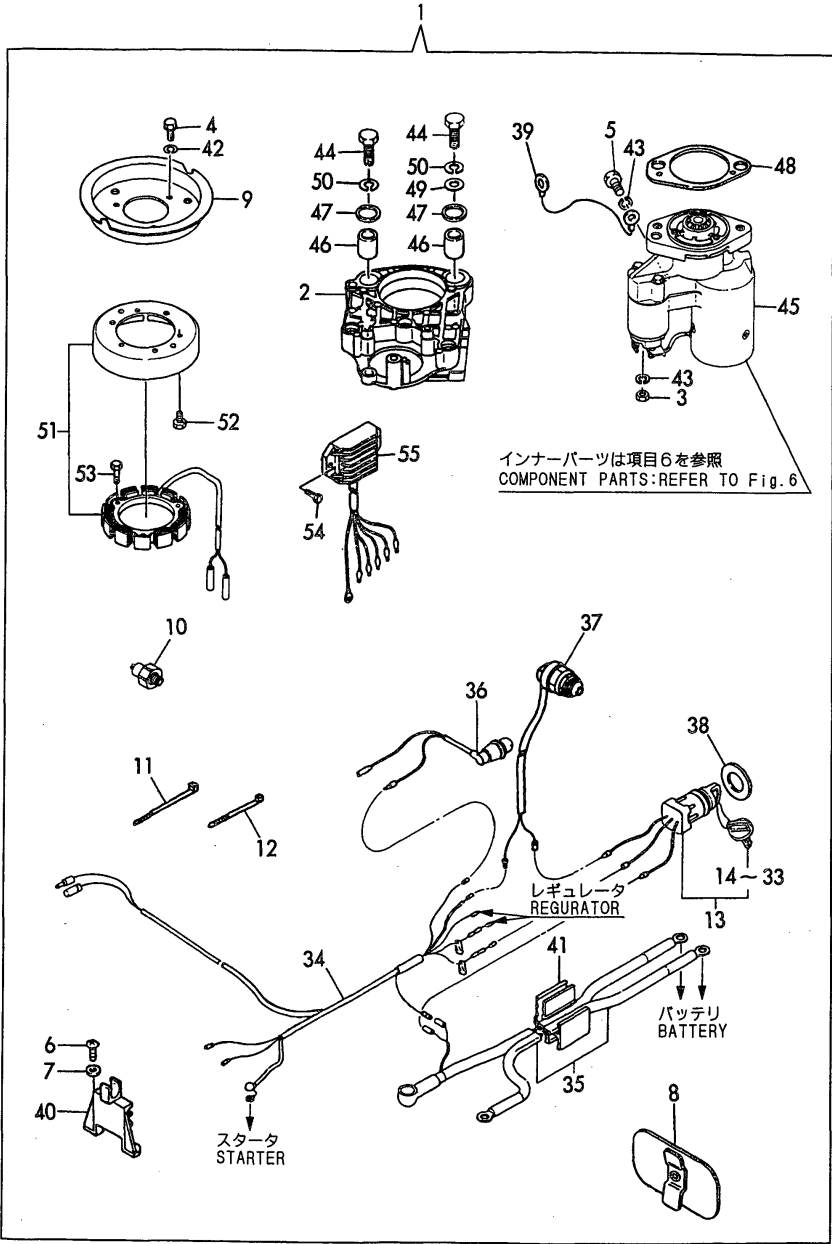
Fig.37 電気改装 (オプション) ELECTRIC REMODELING (OPTIONAL)
