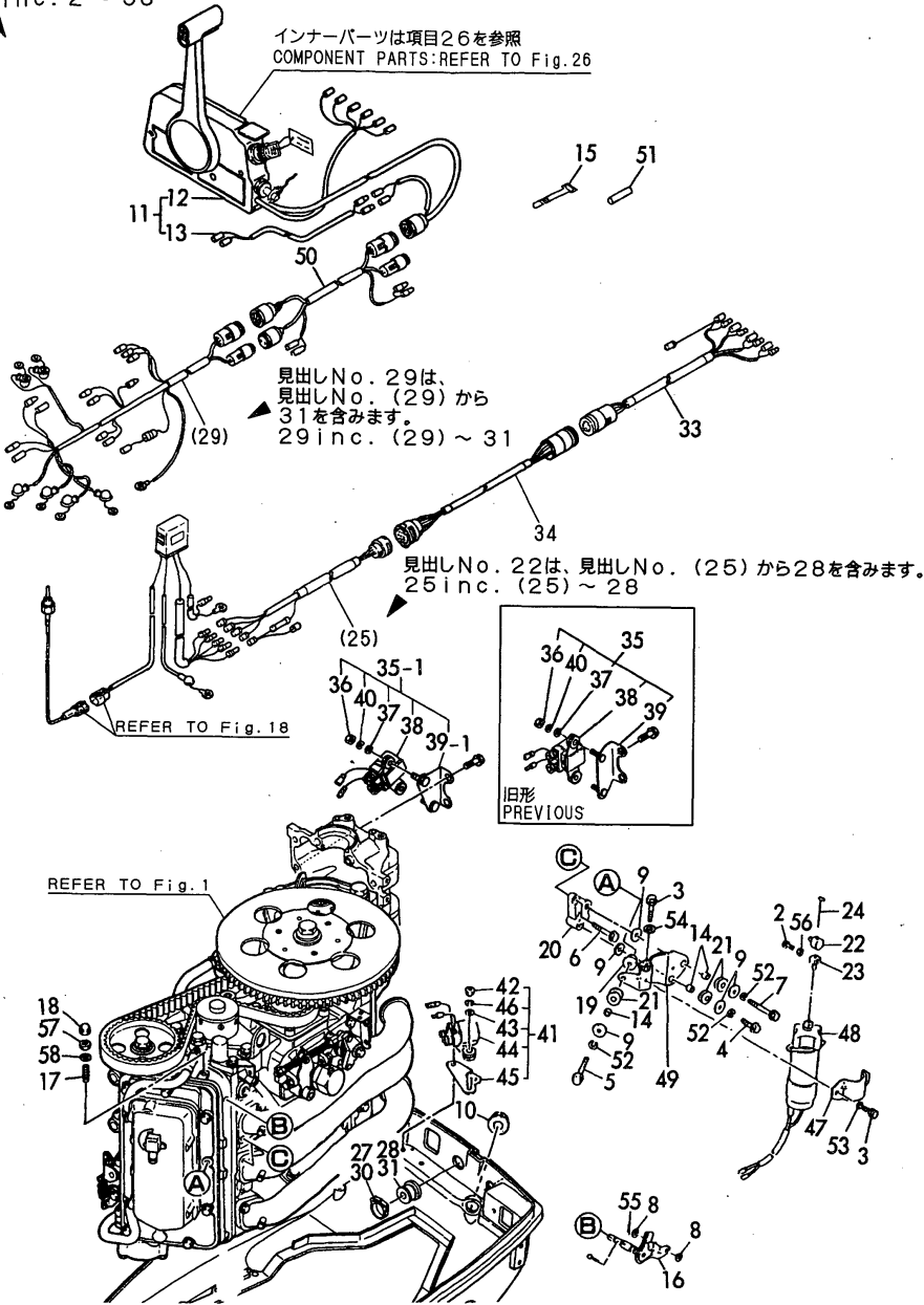
Fig.31 リモコン (タイプC) (オプション) REMOTE CONTROL (TYPE - C) (OPTIONAL)
