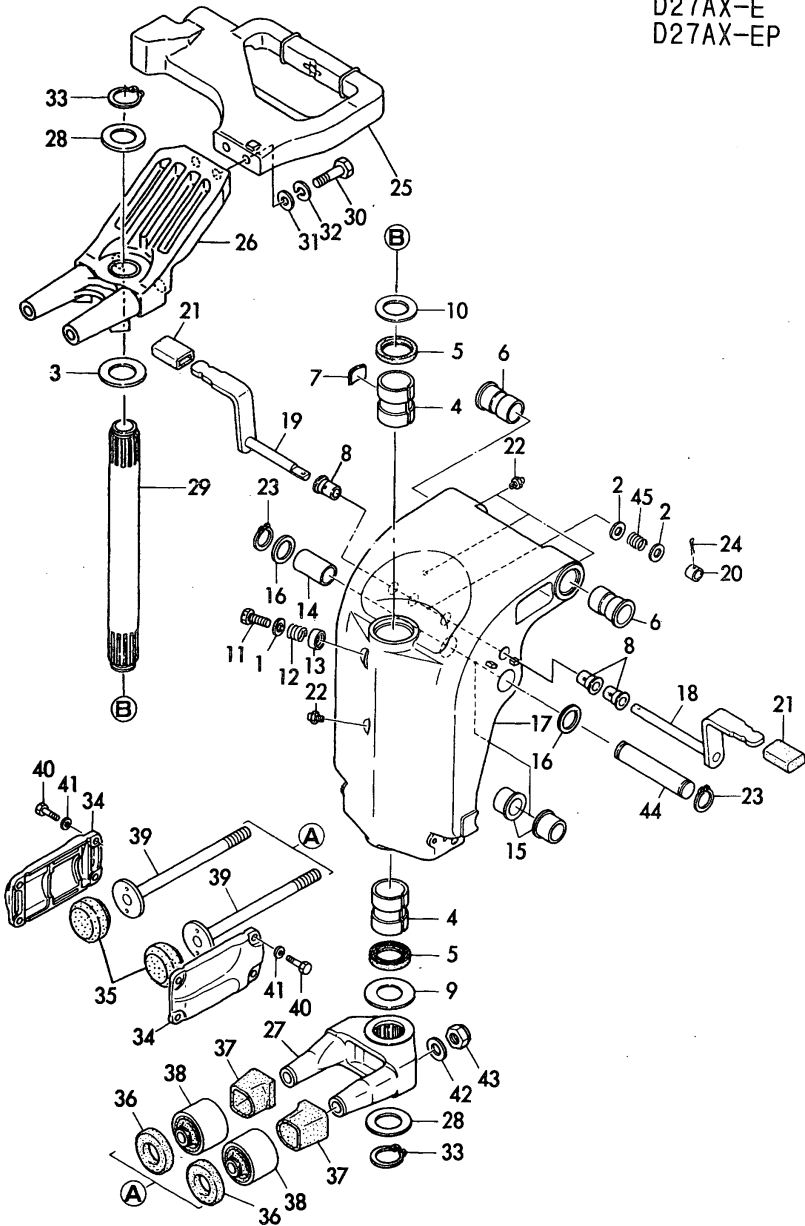
Fig.16 スイベル/ステアリングブラケット SWIVEL/STEERING BRACKET
