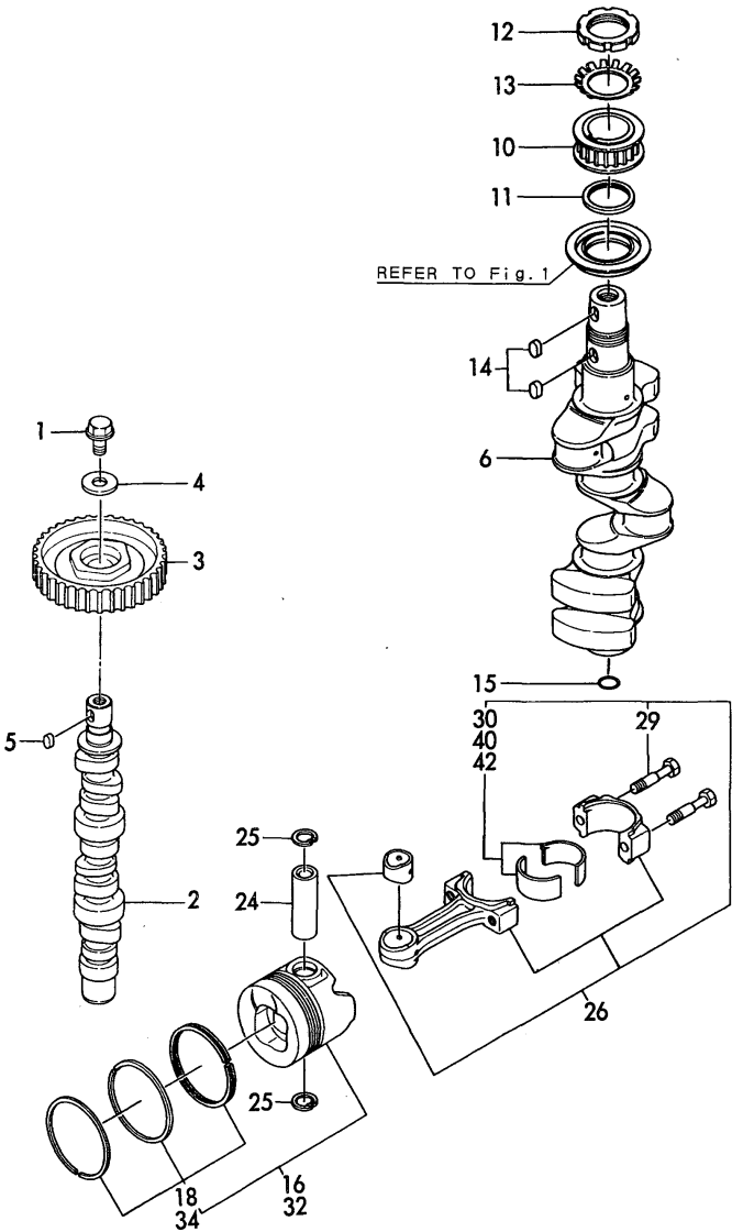
Fig.5 クランクシャフト&ピストン CRANK SHAFT & PISTON
