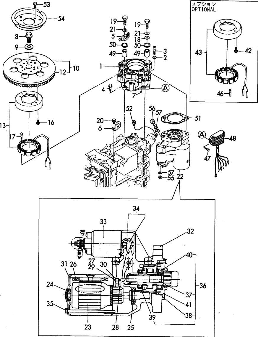
Fig.6 フライホイール、スタータ&ジェネレータ FLYWHEEL, STARTER & GENERATOR
