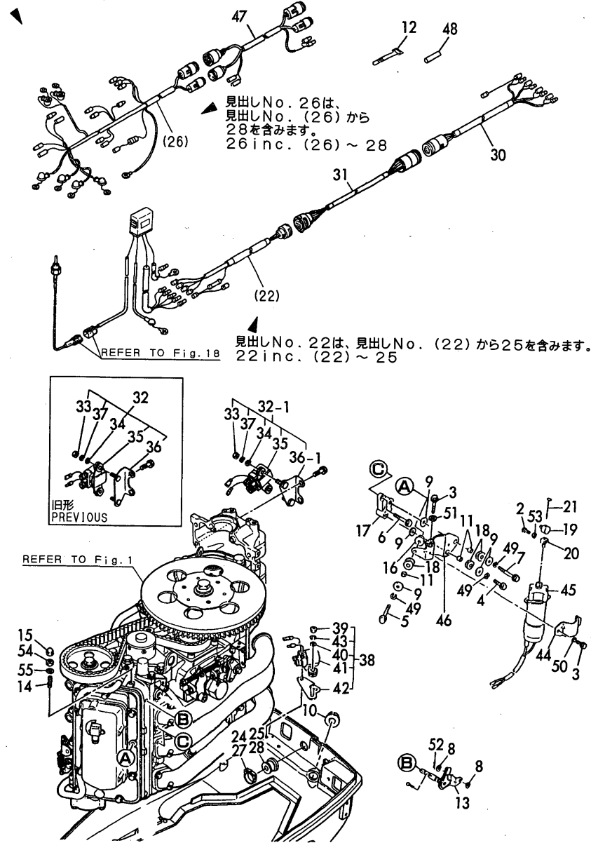
Fig.30 リモコン (タイプB) (オプション) REMOTE CONTROL (TYPE-B) (OPTIONAL)
