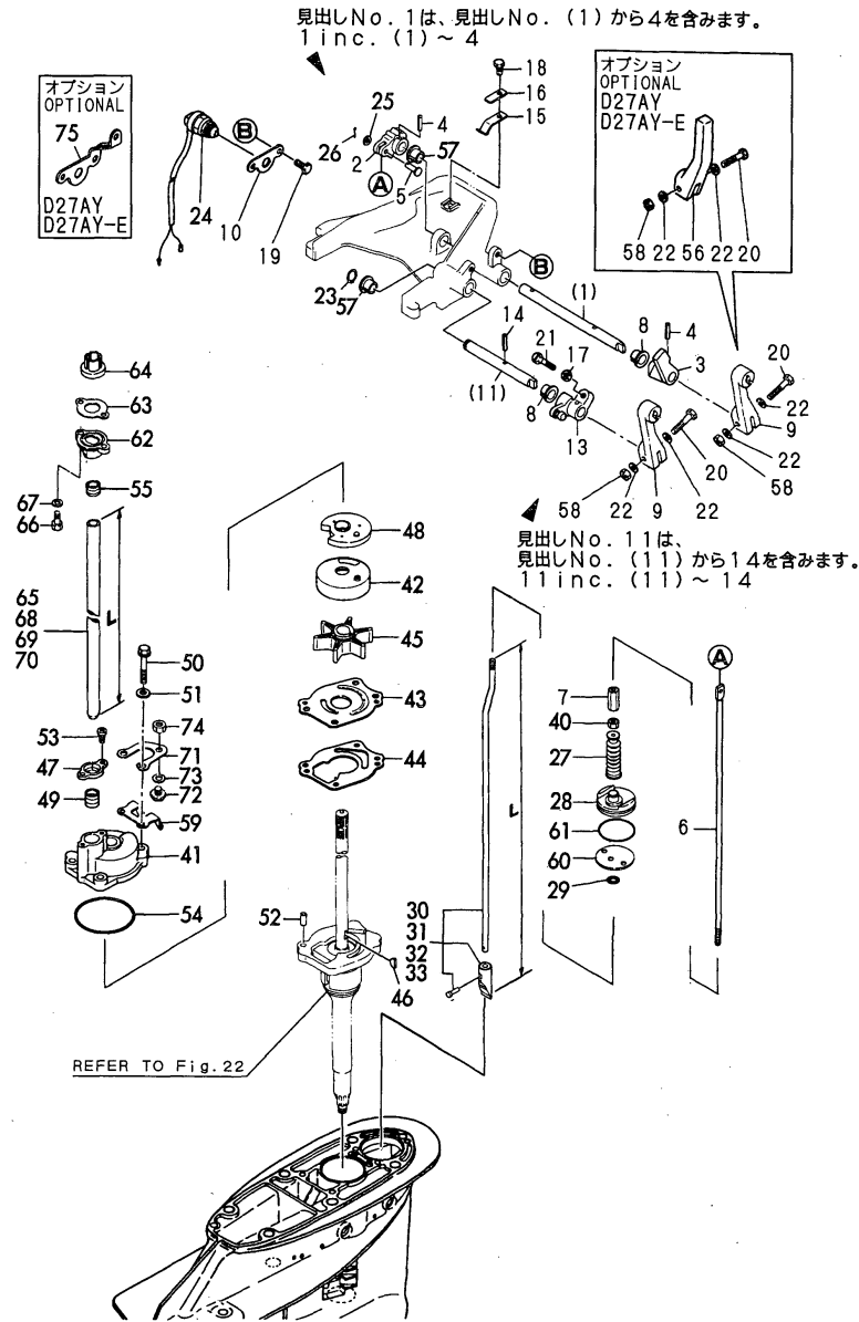
Fig.21 シフト装置&冷却水ポンプ SHIFT DEVICE & COOLING WATER PUMP
