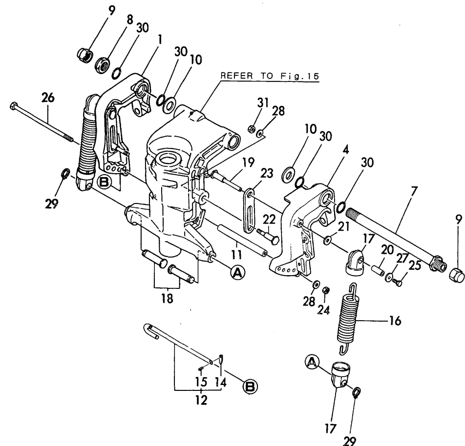
Fig.12 クランプブラケット CLAMP BRACKET
