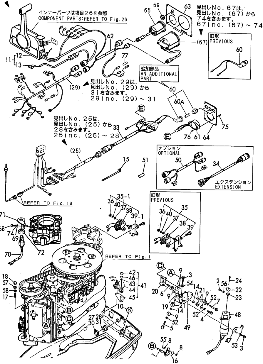
Fig.32 リモコン (タイプD) (オプション) REMOTE CONTROL (TYPE-D) (OPTIONAL)
