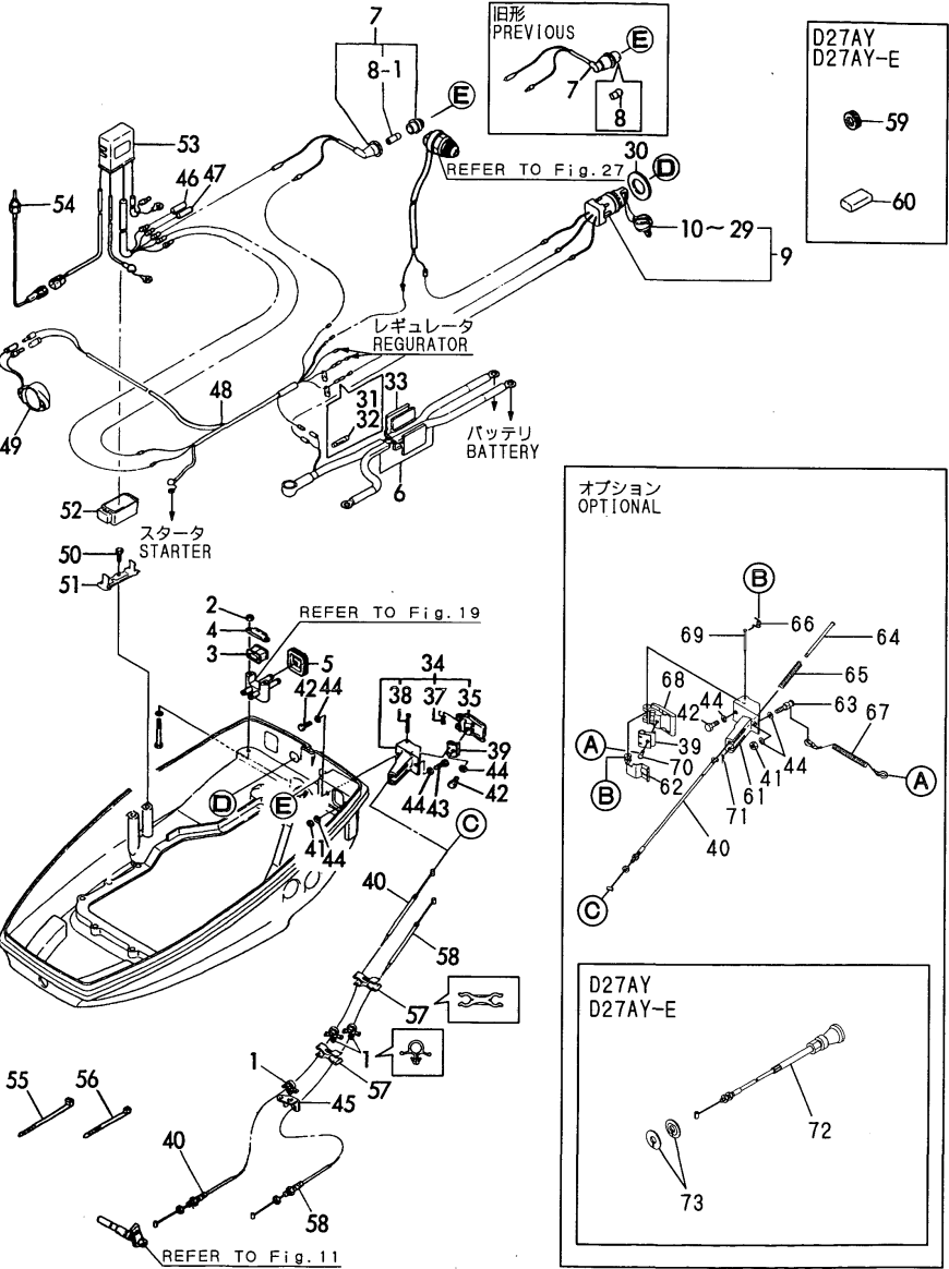
Fig.18 ストップレバー&ロフセット部品 STOP LEVER & LOWER SET PART
