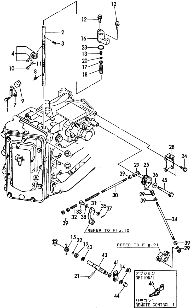
Fig. 11 エンジンコントロール装置 ENGINE CONTROL DEVICE
