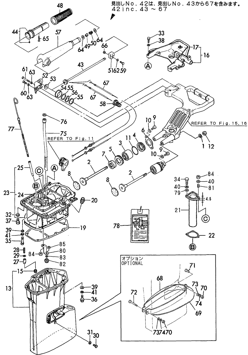
Fig.20 ステアリングハンドル&アッパーケース STEERING HANDLE & UPPER HOUSING
