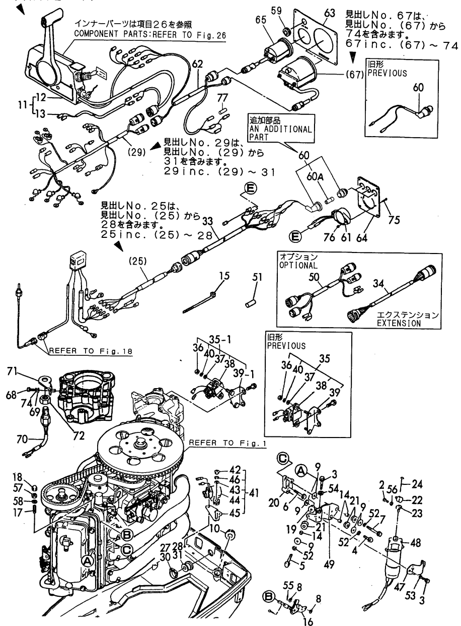
Fig. 32 リモコン (タイプD) (オプション) REMOTE CONTROL (TYPE-D) (OPTIONAL)
