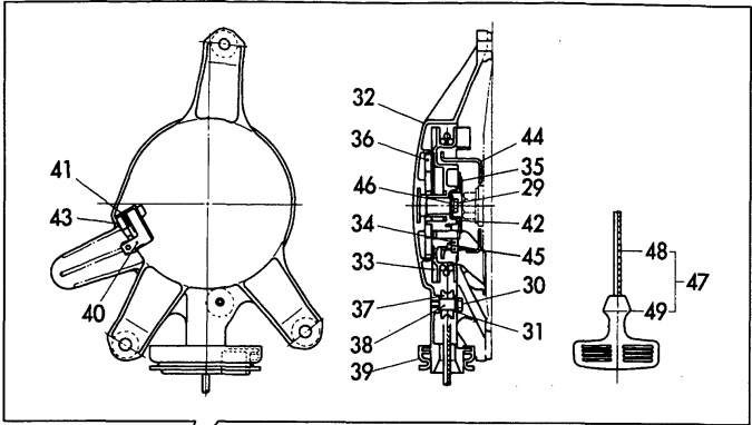
Fig.7 フライホイール&リコイルスタータ FLYWHEEL & RECOIL STARTER
