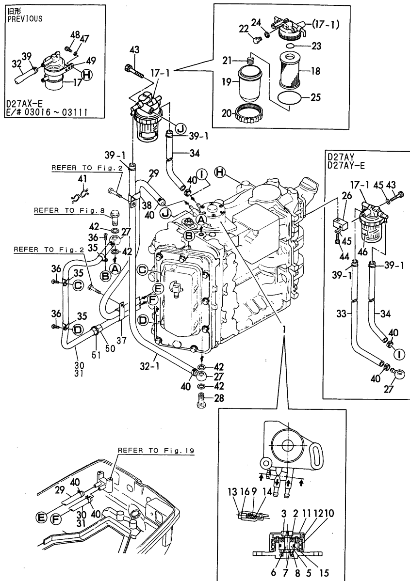
Fig. 9 燃料フィルタ&燃料パイプ FUEL STRAINER & FUEL PIPE
