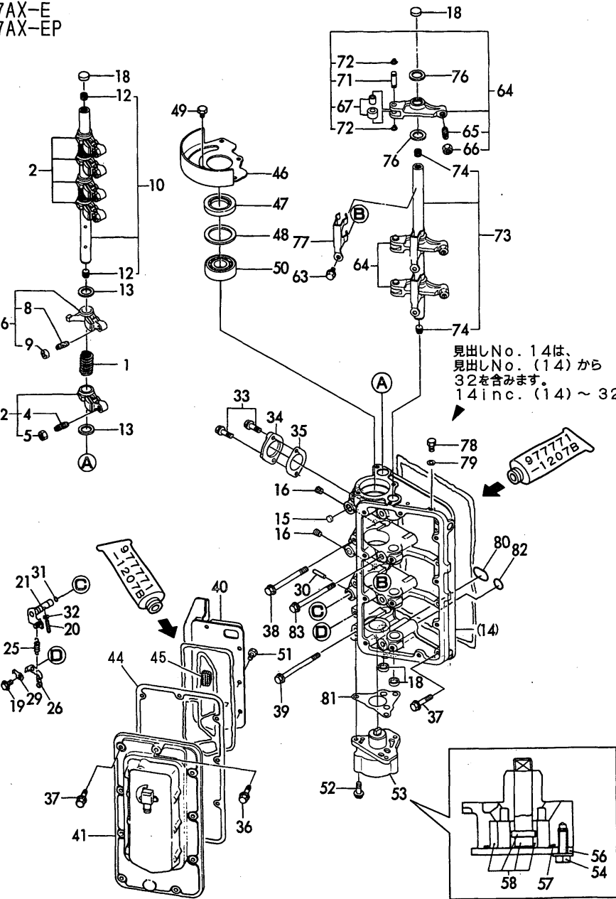
Fig.3 ボンネット & 潤滑油ポンプ BONNET & LUB.OIL PUMP
