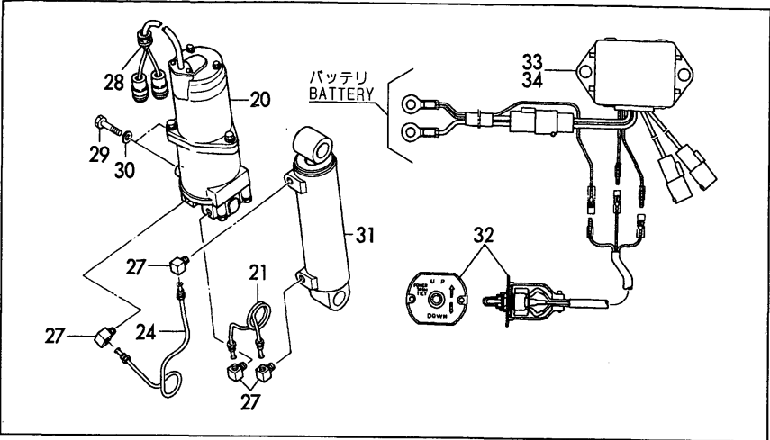
Fig.13 クランプブラケット CLAMP BRACKET
