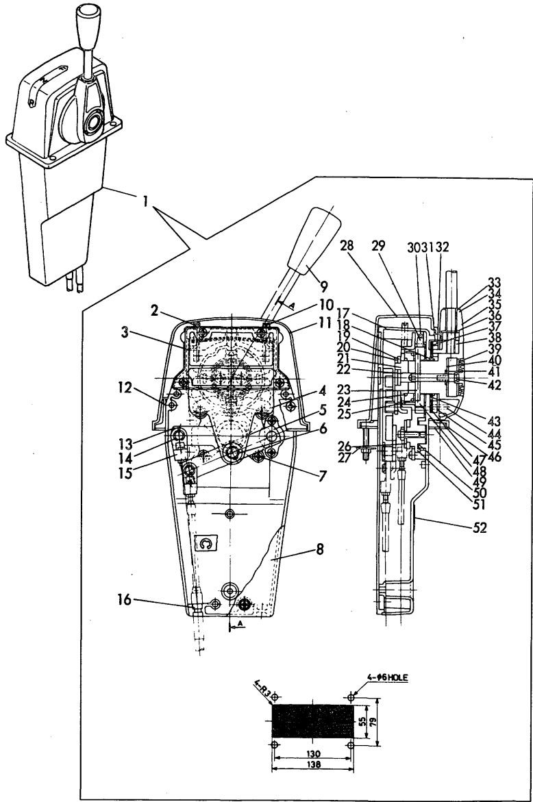
Fig.33 KLトップコントロール (オプション) KL TOP CONTROL (OPTIONAL)
