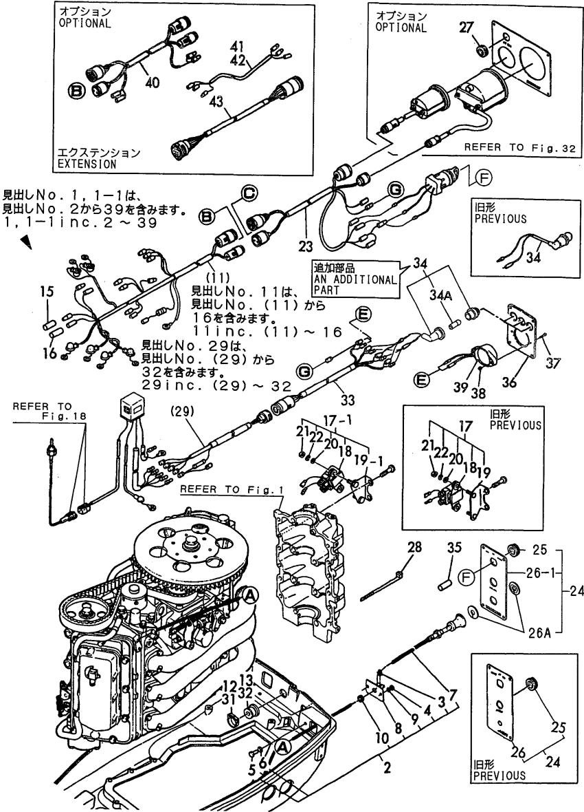
Fig.29 リモコン (タイプA) (オプション) REMOTE CONTROL (TYPE-A) (OPTIONAL)
