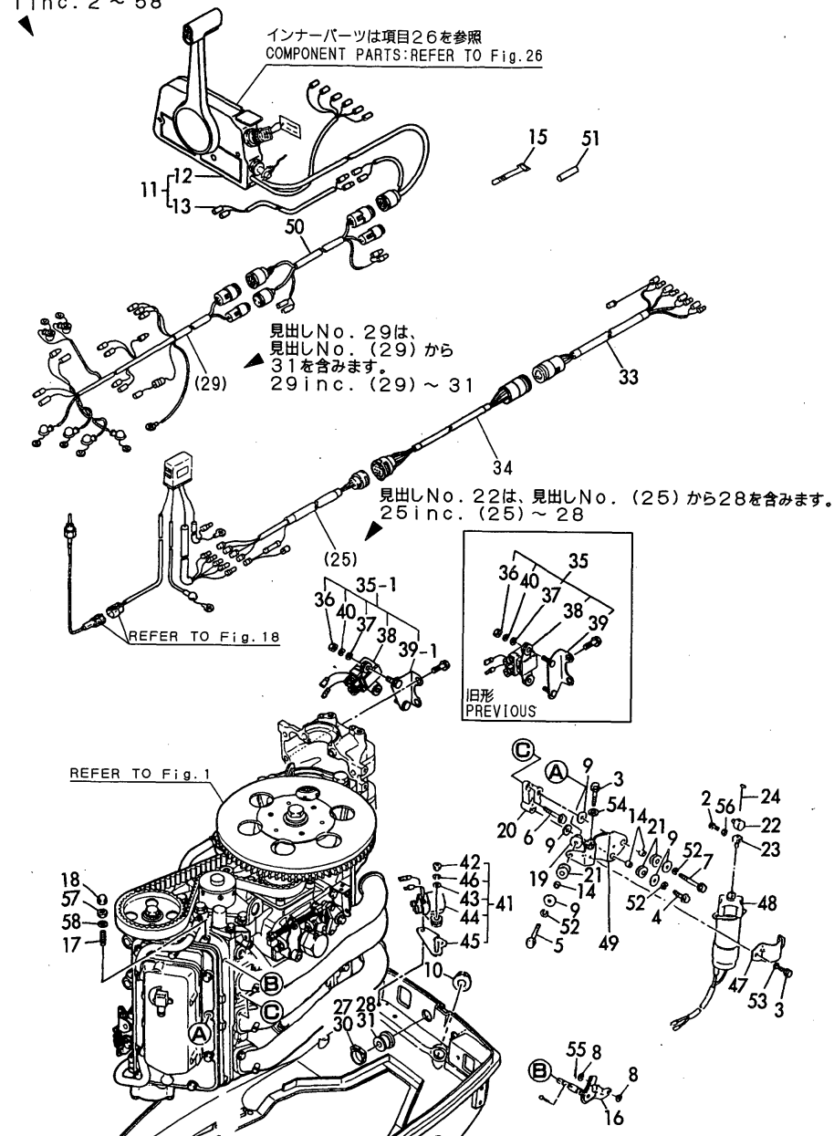
Fig. 31 リモコン (タイプC) (オプション) REMOTE CONTROL (TYPE - C) (OPTIONAL)
