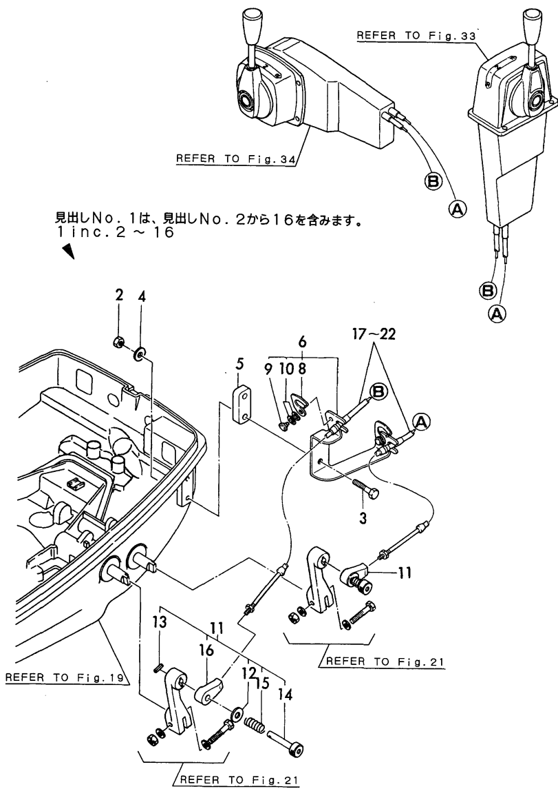
Fig.23 シフトリモコン SHIFT REMOTE CONTROL
