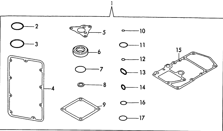
Fig.35 パッキンセット (オプション) GASKET SET (OPTIONAL)
