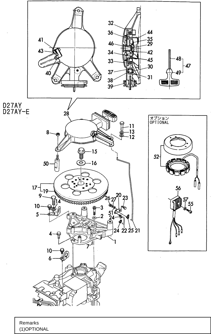
Fig.7 フライホイール&リコイルスタータ FLYWHEEL & RECOIL STARTER
