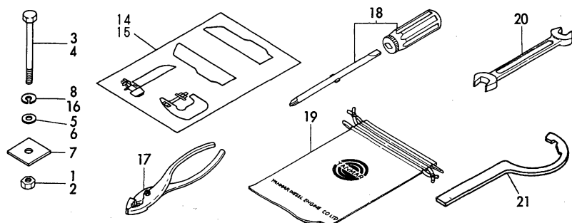
Fig. 25 工具&スペアパーツ TOOL & SPARE PART
