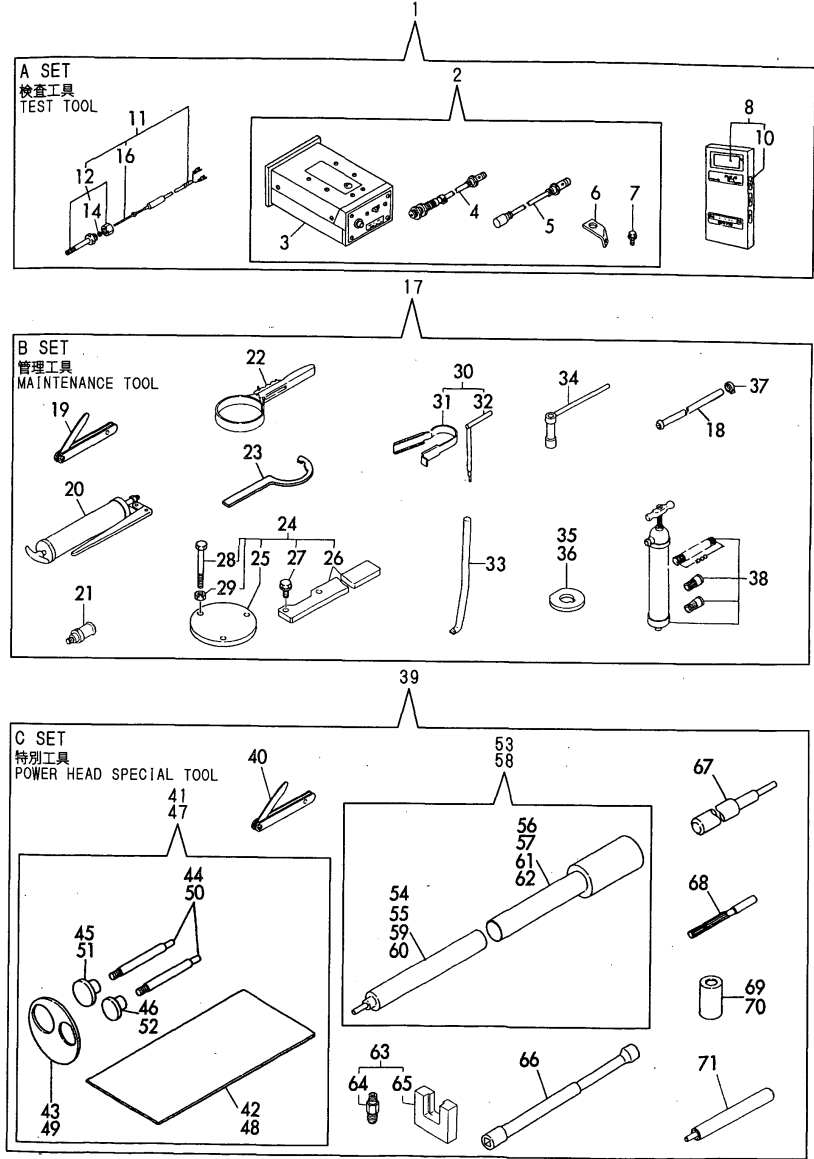
Fig.27 特殊工具(1)(オプション) SPECIAL TOOL(1)(OPTIONAL)
