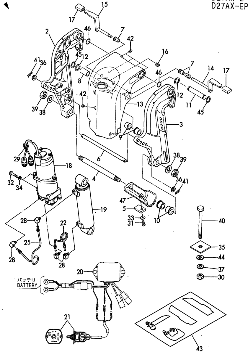
Fig.36 パワーチルト (オプション) POWER TILT (OPTIONAL)
