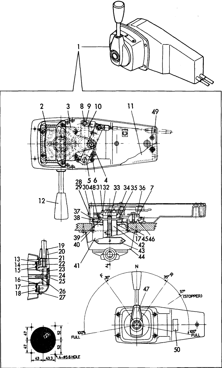
Fig.34 KLサイドコントロール (オプション) KL SIDE CONTROL (OPTIONAL)
