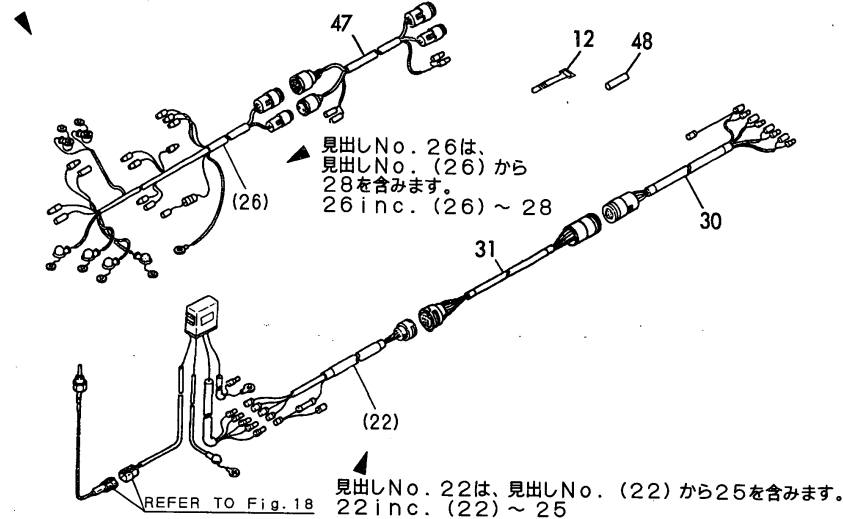
Fig.30 リモコン (タイプB) (オプション) REMOTE CONTROL (TYPE-B) (OPTIONAL)
