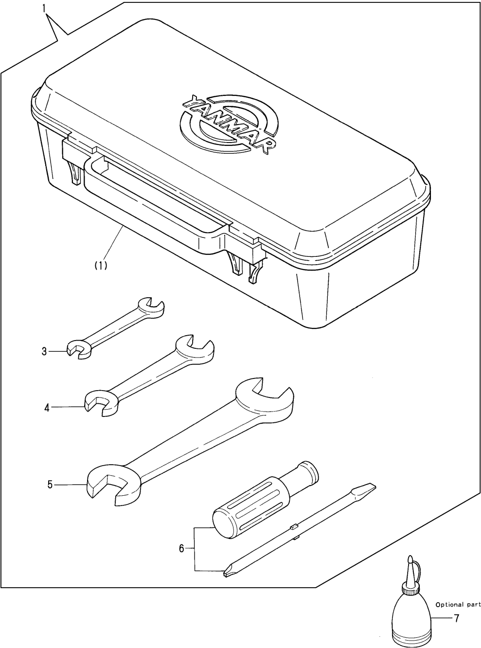
Fig.55.TOOL
