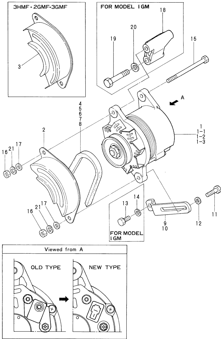
Fig.47.GENERATOR(AC)
